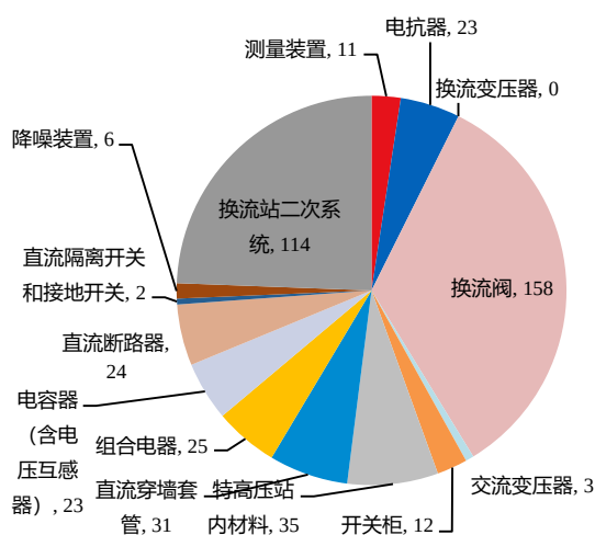
图表 3 格尔木±400 千伏换流站扩建工程设备采购情况（百万元）
