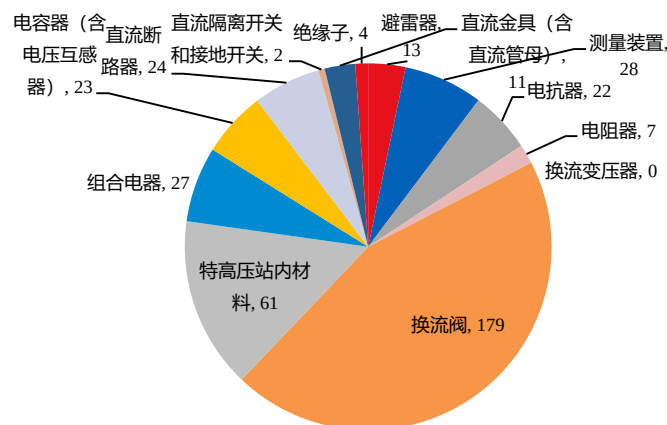
图表 4 拉萨±400 千伏换流站扩建工程设备采购情况（百万元）
