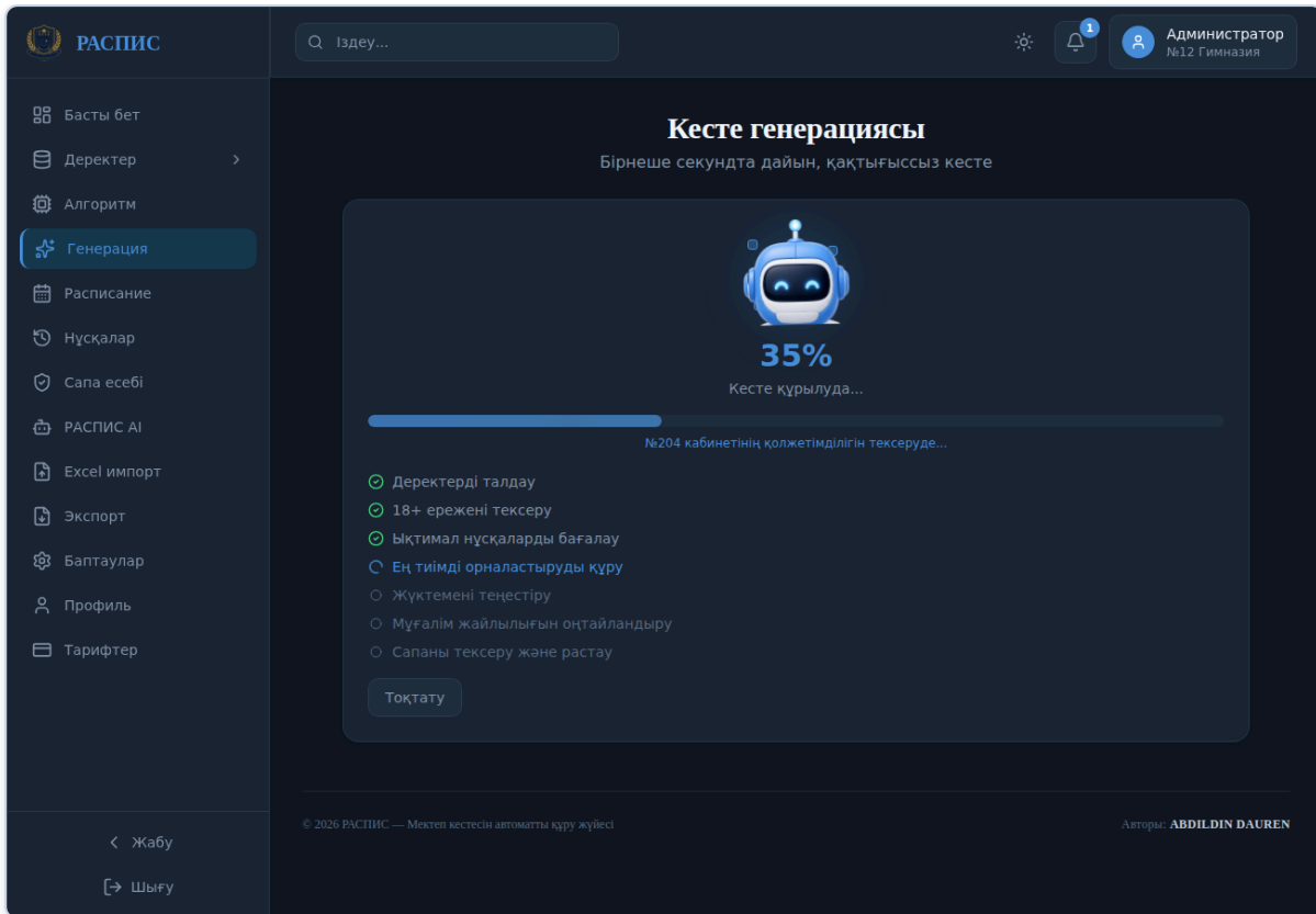
16-сурет. Генерация барысы: кезеңдер және тірі күй жолы
