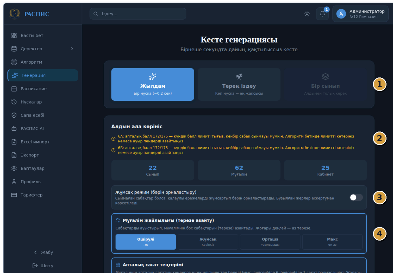
14-сурет. Генерация беті: режимдер мен параметрлер
