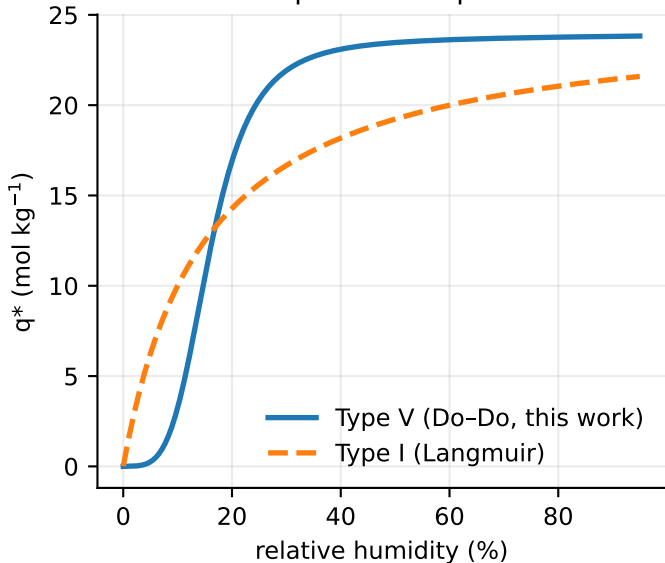
A. Equilibrium uptake
