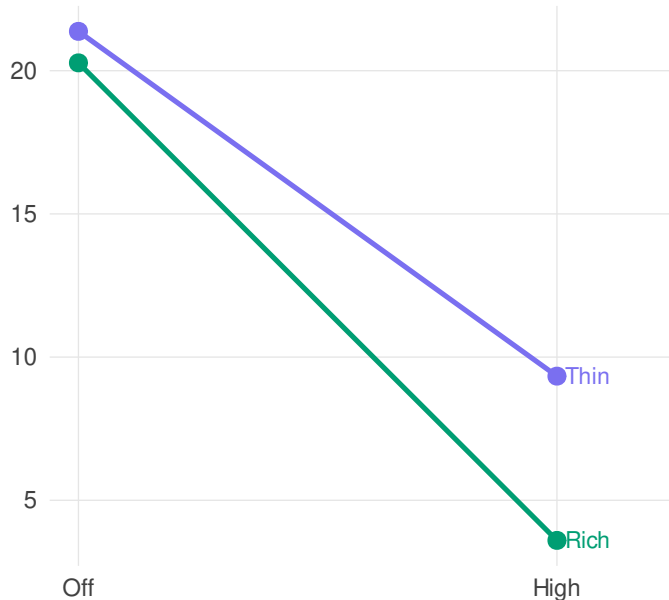
Hard population MAE
