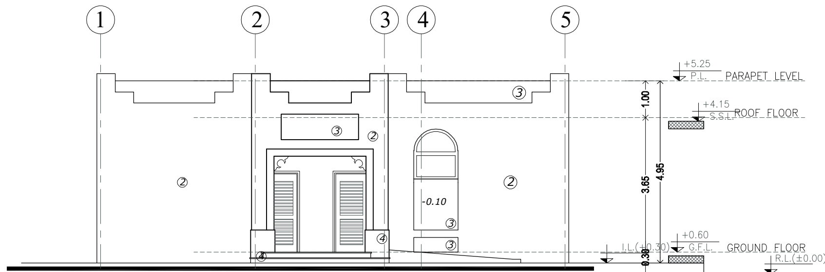
ELEVATION - A
