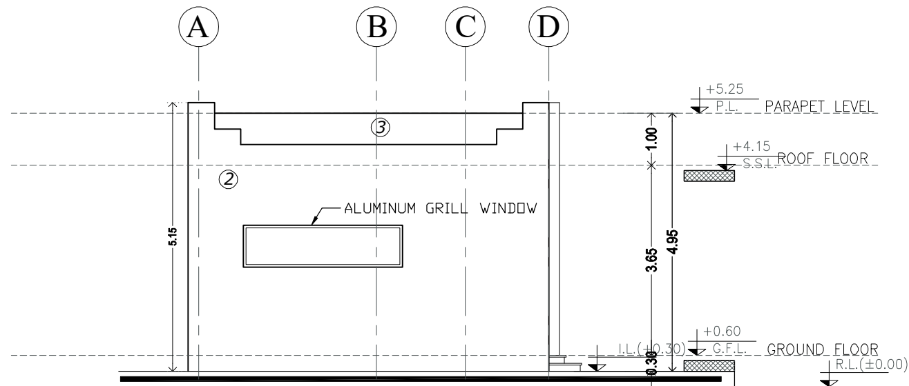
ELEVATION - D
