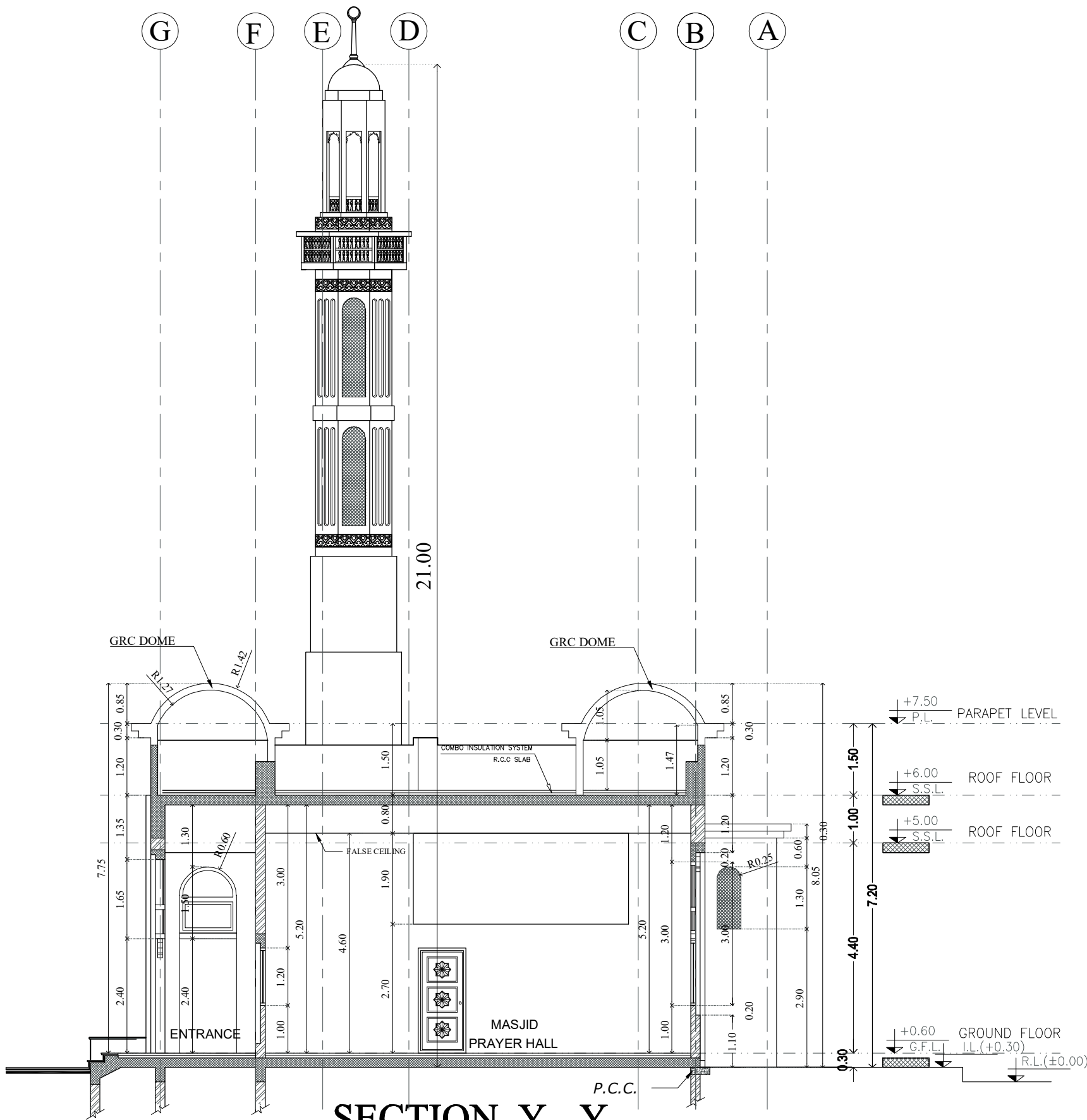
SECTION Y - Y
