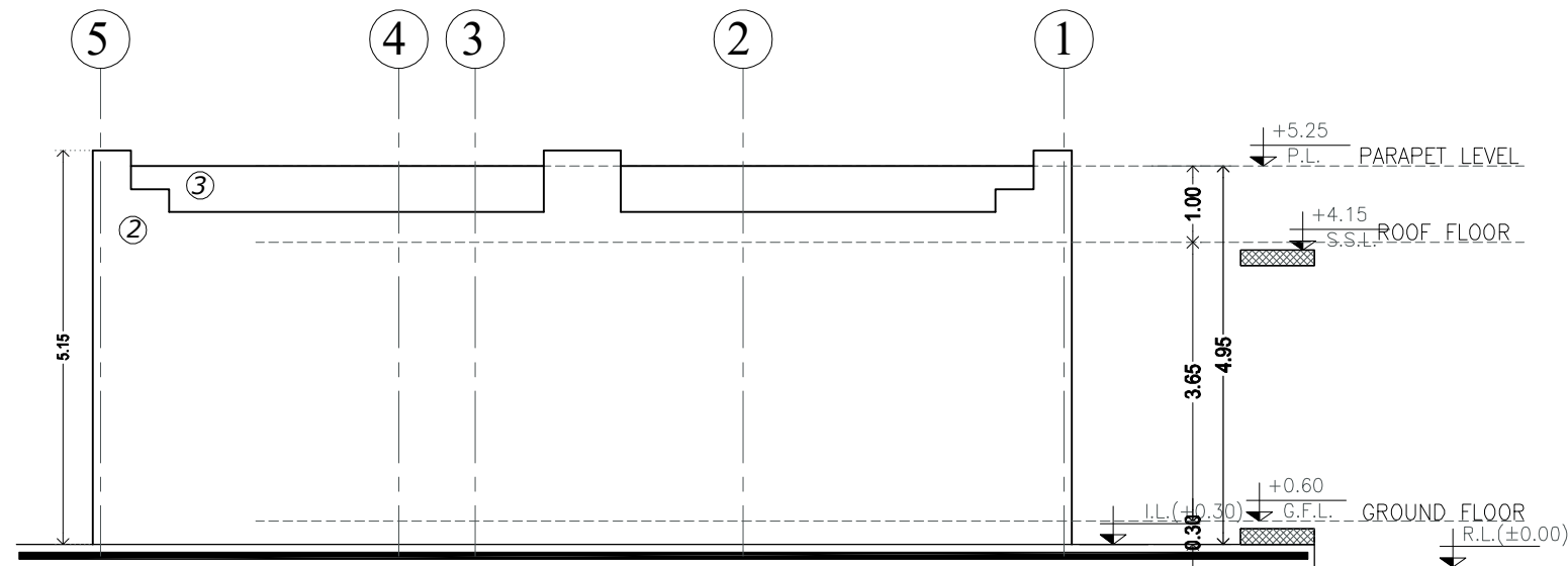
ELEVATION - C
