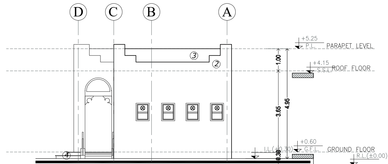
ELEVATION - B
