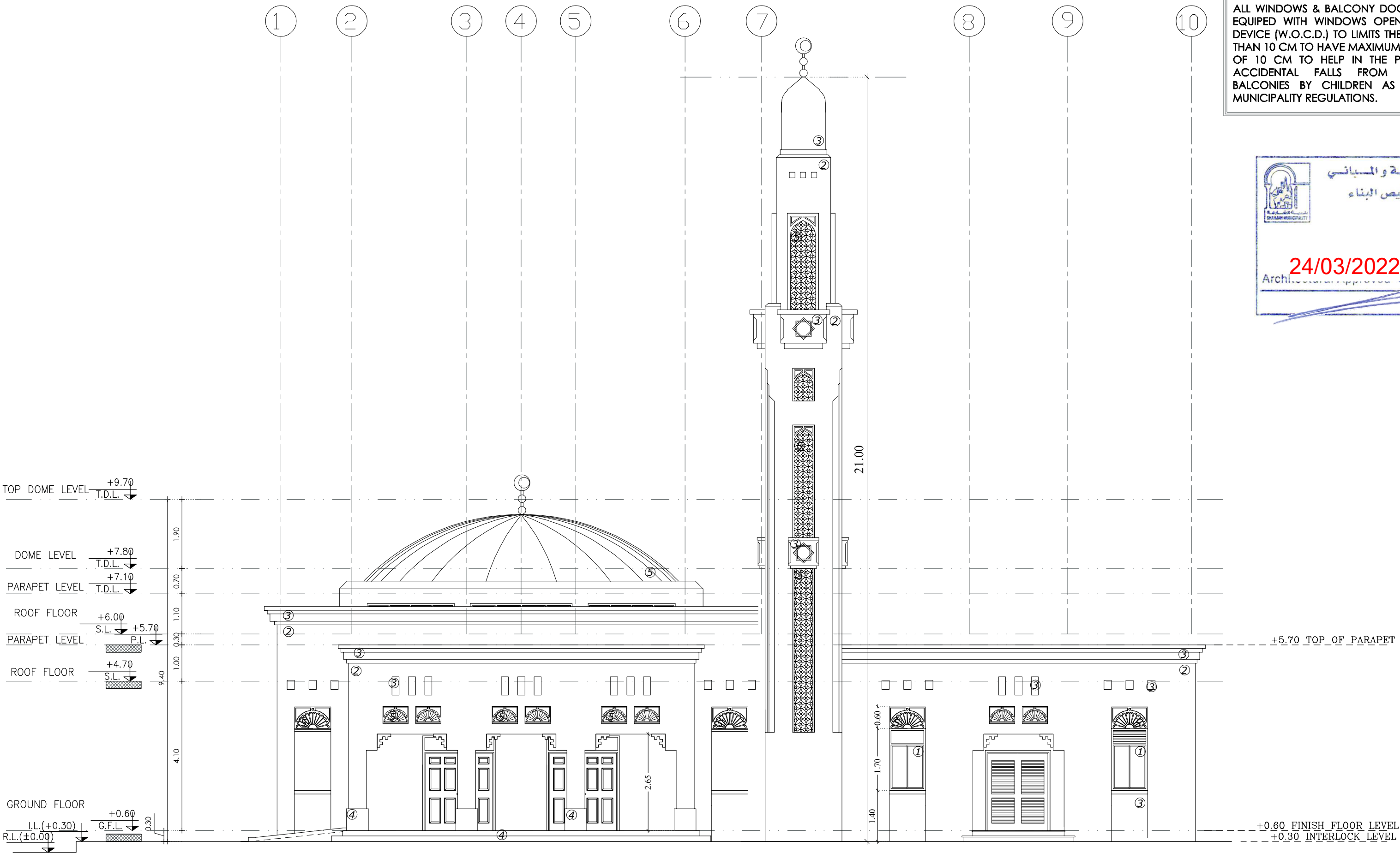
ELEVATION -A
