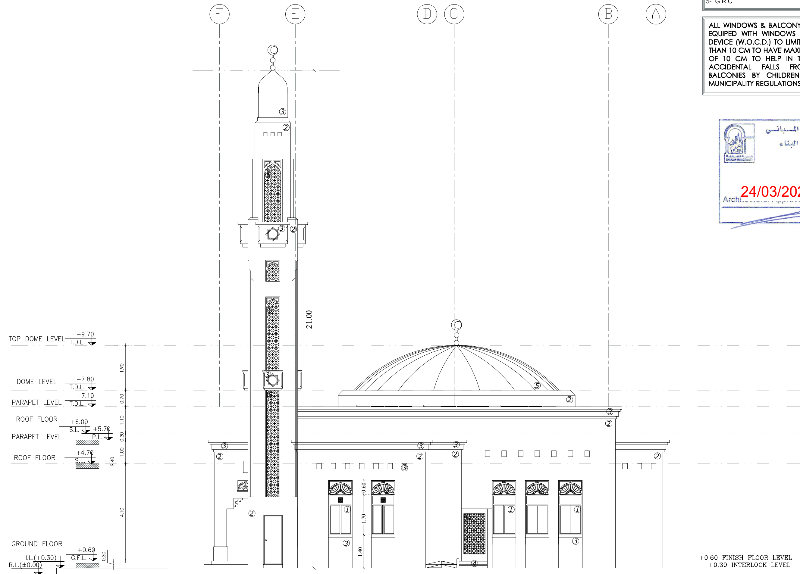
ELEVATION -B
