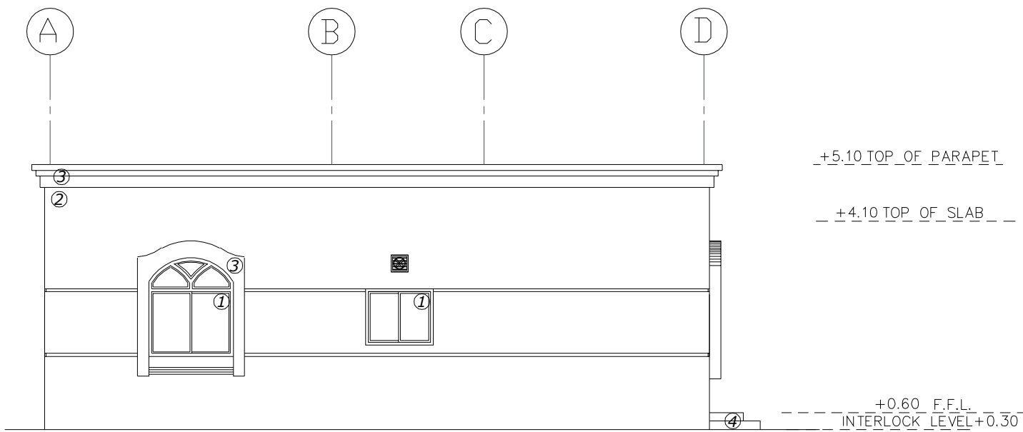
ELEVATION -D (SCALE = 1 : 100)
