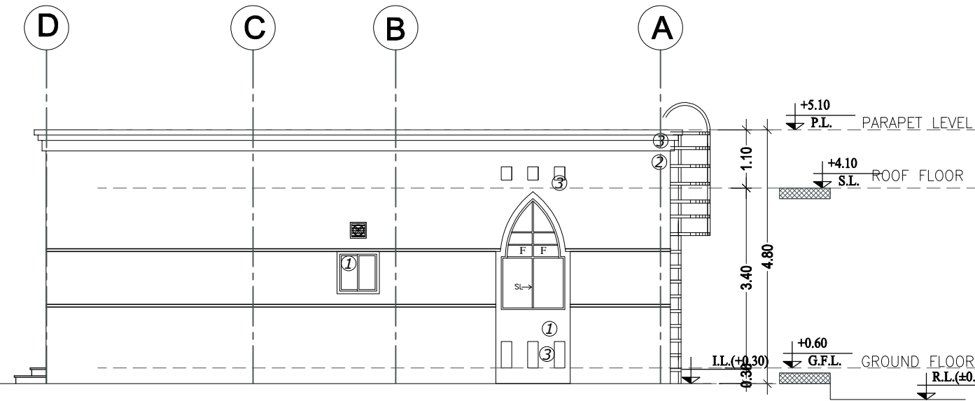
ELEVATION -B
