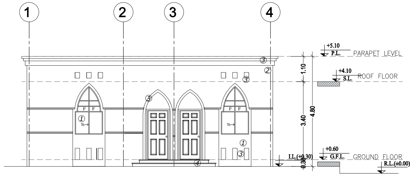
ELEVATION -A
