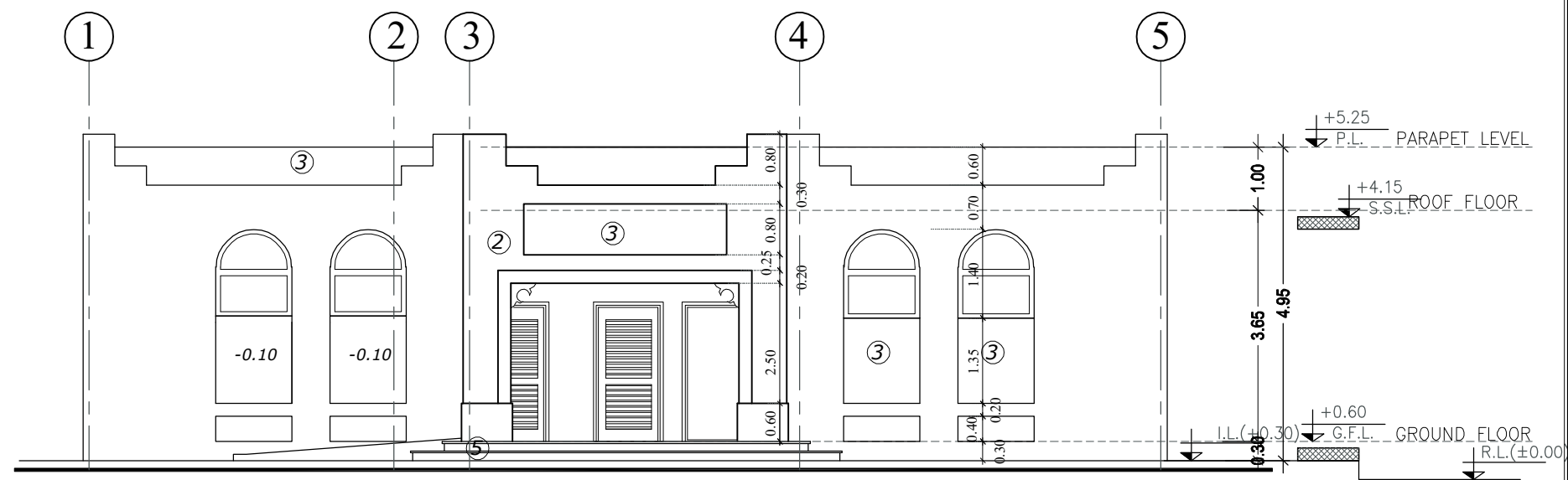
ELEVATION - B
