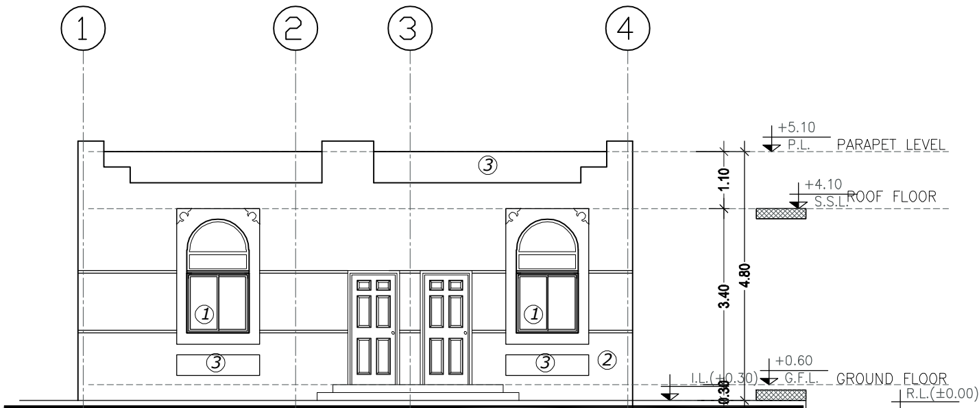
ELEVATION - A
