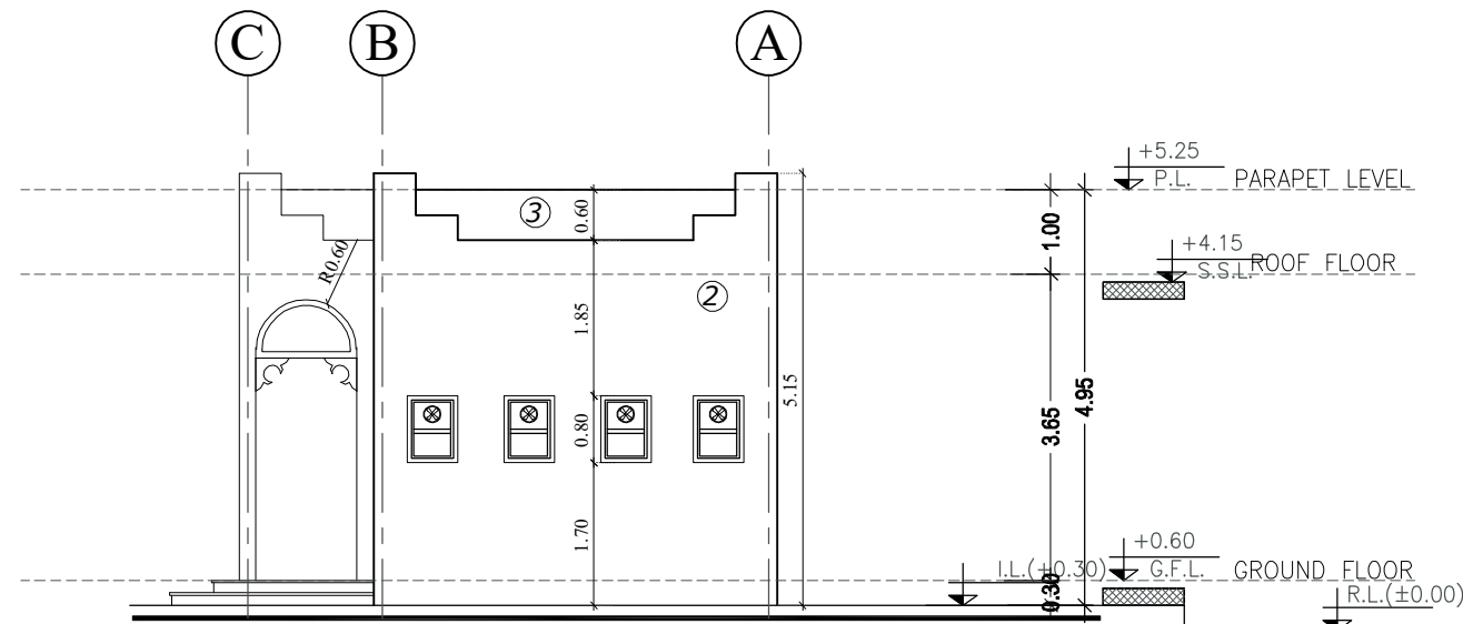
ELEVATION - C
