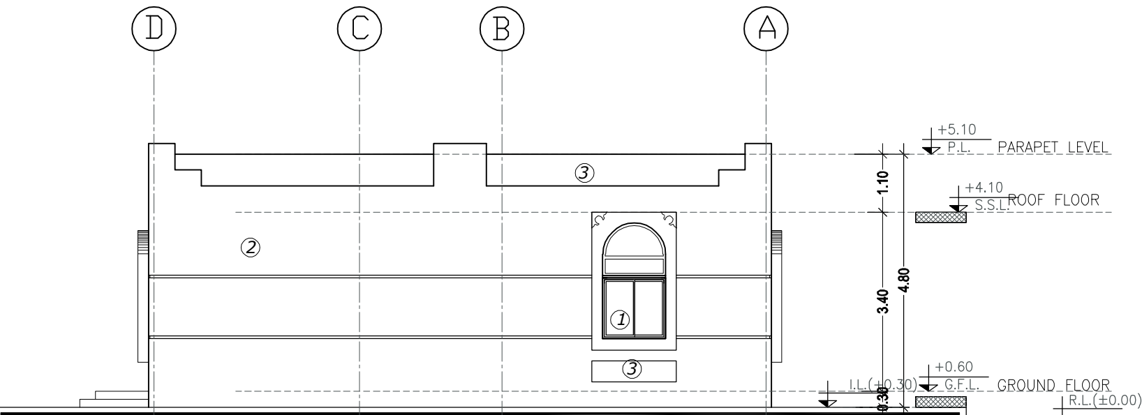
ELEVATION - B
