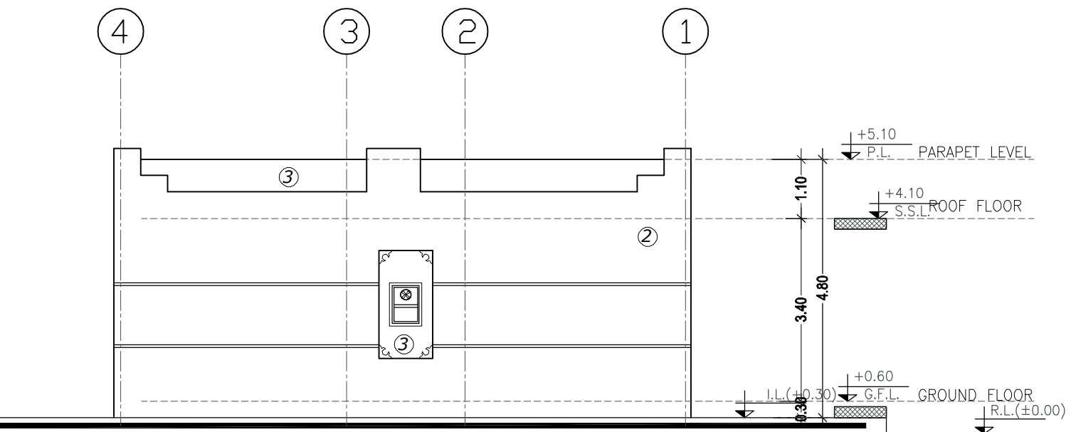
ELEVATION - C
