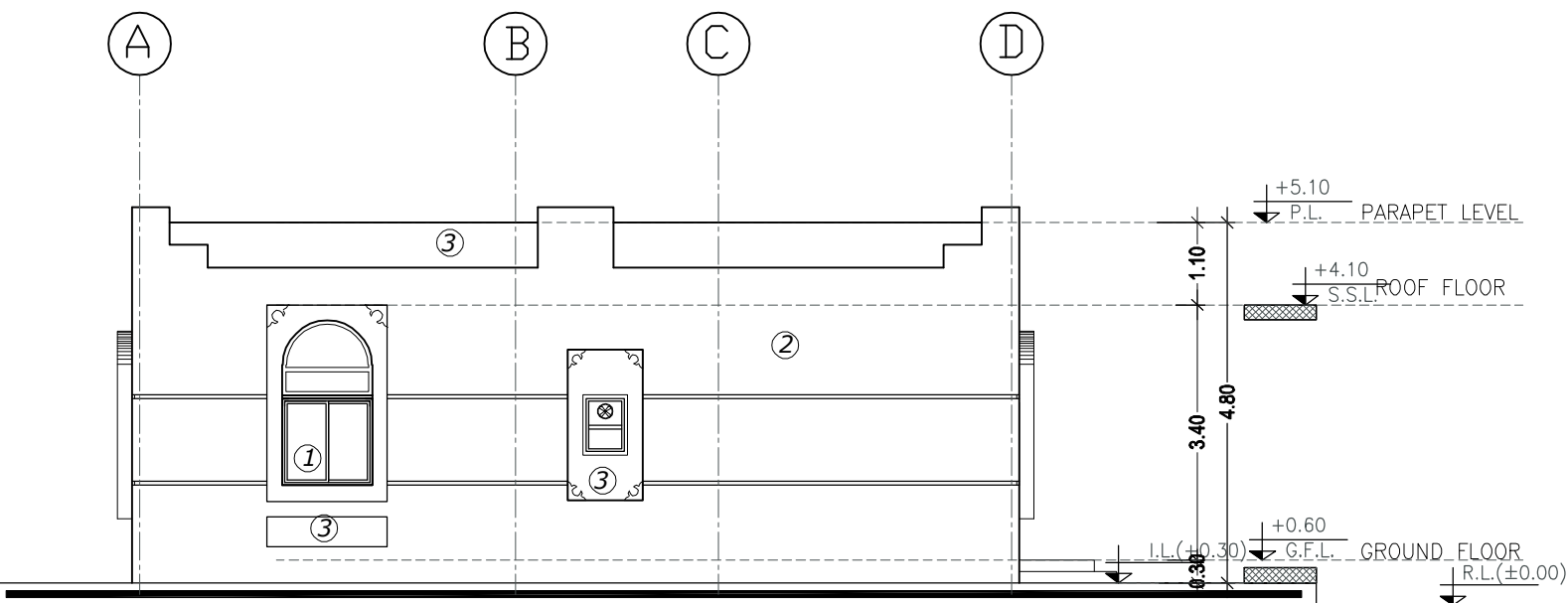
ELEVATION - D
