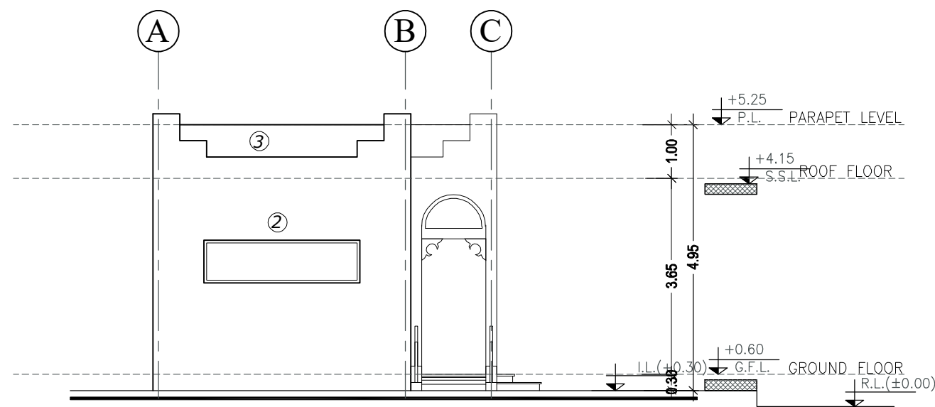
ELEVATION - A
