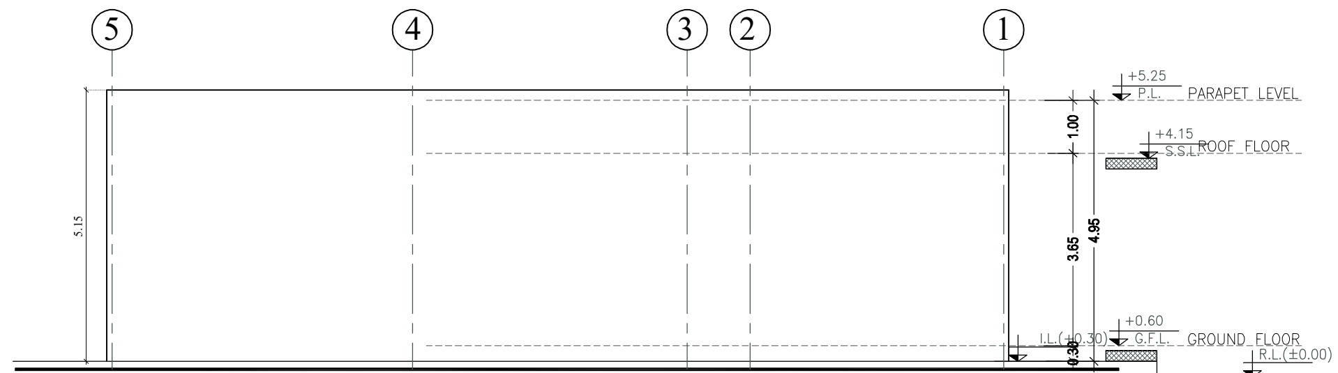
ELEVATION - D
