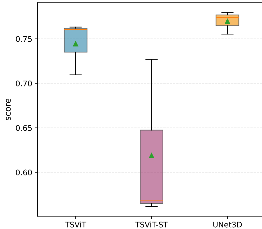
F1 Score
