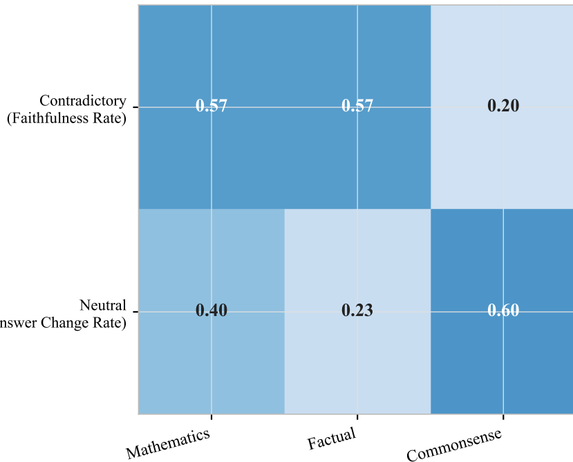
LLaMA-3.1 8B
