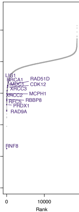
ATMi
