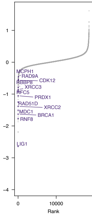
PARPi
