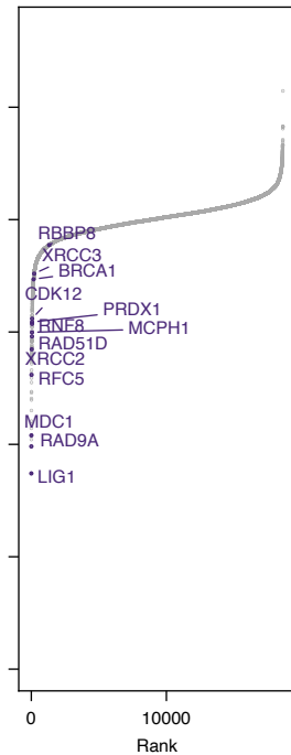
ATRi
