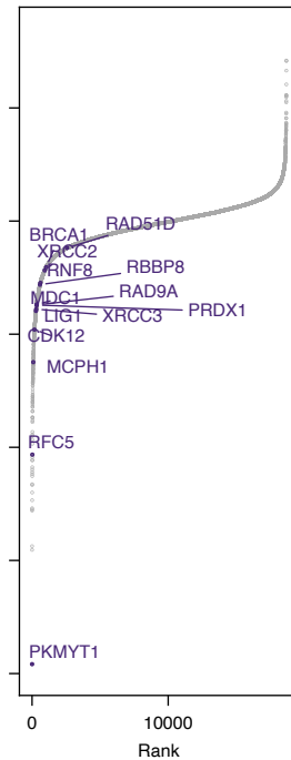
WEE1i
