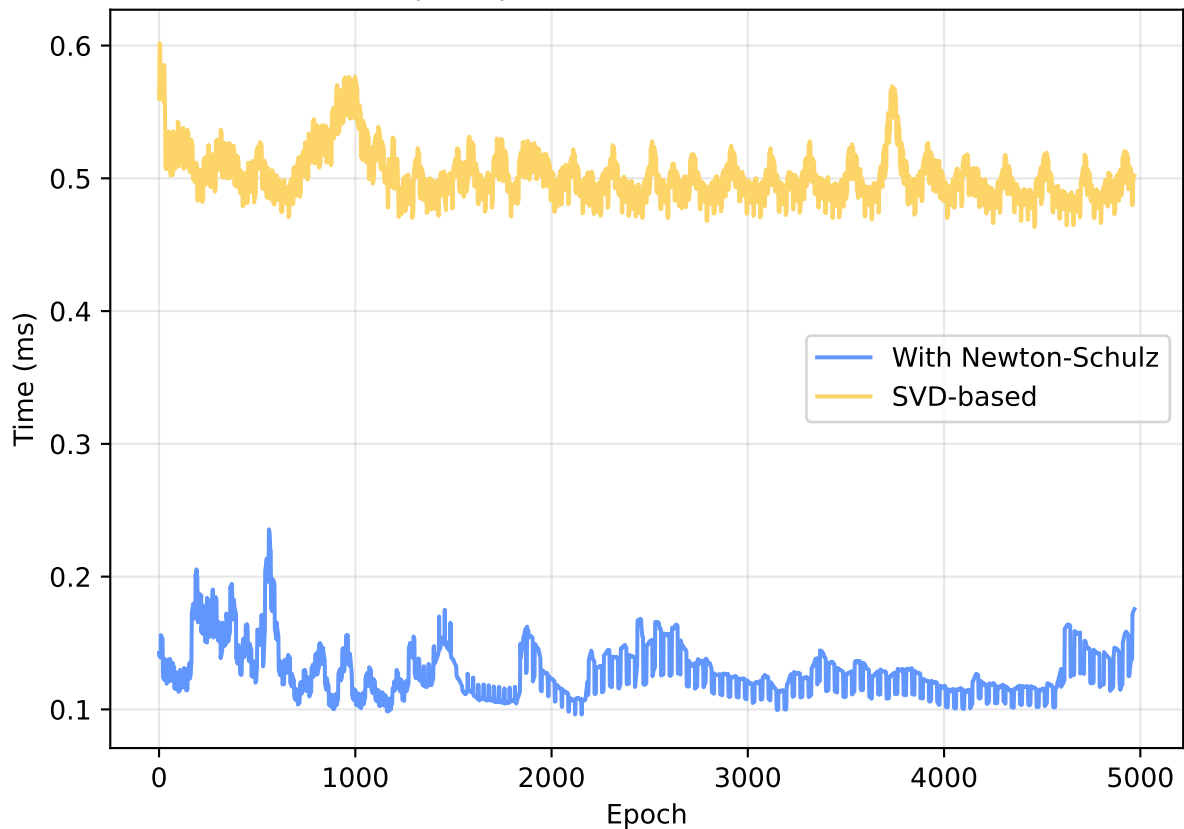
Time per Epoch - Newton-Schulz vs SVD
