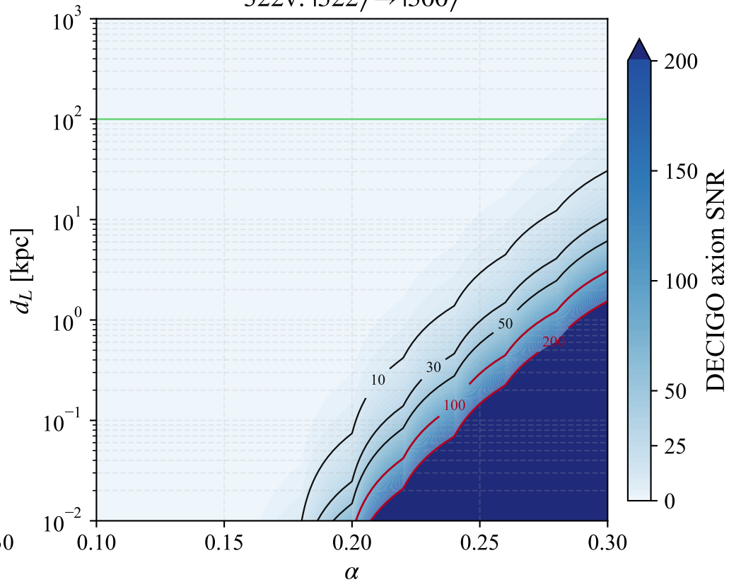
322v: |322\rangle \rightarrow |300\rangle
