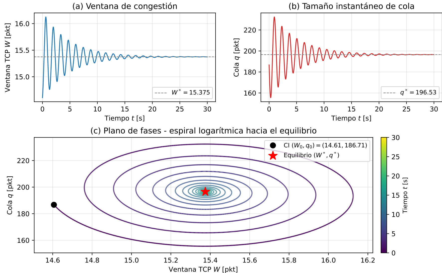
Fig. 2 - Régimen estable: convergencia al equilibrio ( w_q = 0.05 , perturbación inicial del 5%)
