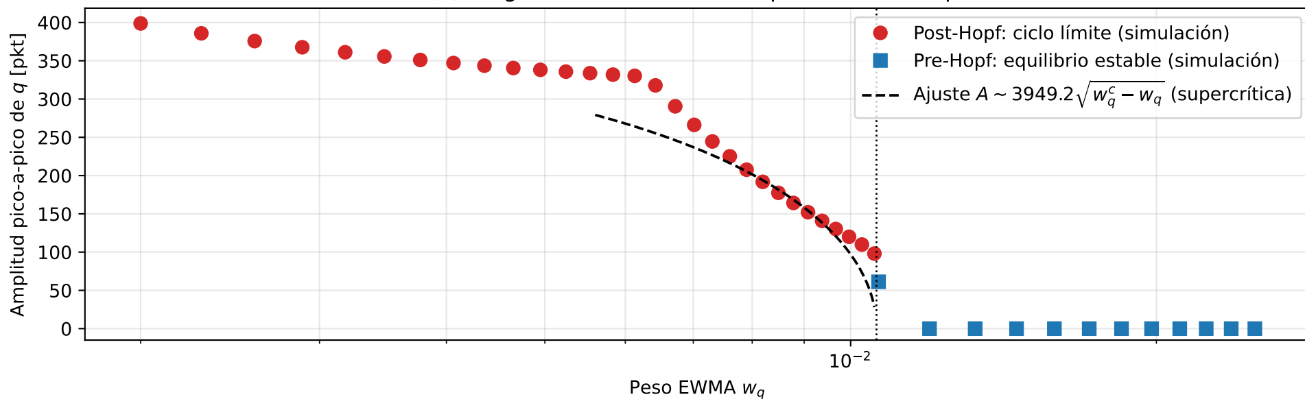
(d) Diagrama de bifurcación supercrítica de Hopf
