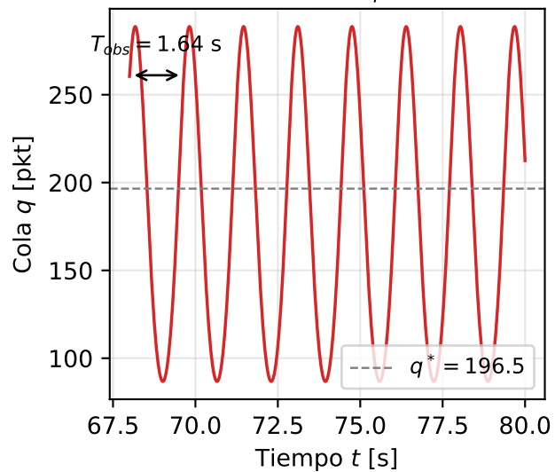
(a) Ciclo límite: q(t) , w_q = 0.008 (zoom)
