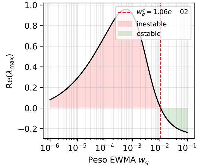
(c) Análisis lineal
