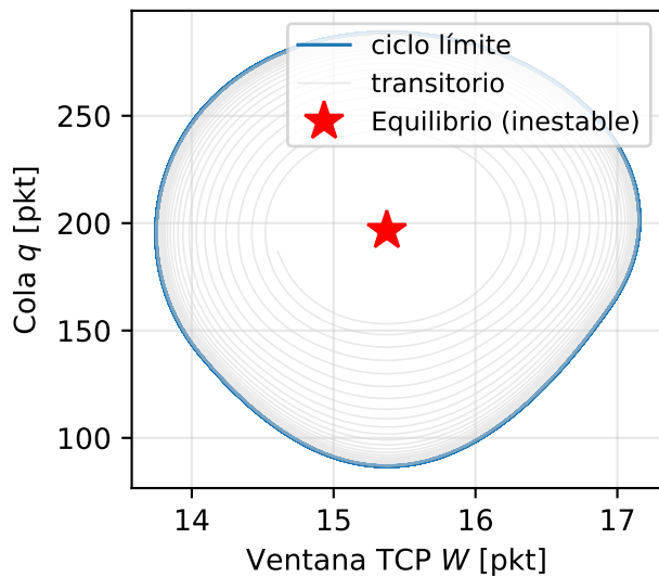
(b) Plano de fases - ciclo límite
