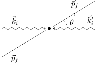
Fig. 1: Situazione cinematica dell'annichilazione elettrone-positrone nel sistema di riferimento del centro di massa. A causa della conservazione di energia e impulso, \omega_i = \omega'_i = E_f = \bar{E}_f e \vec{k}_i = -\vec{k}'_i , \vec{p}_f = -\vec{p}'_f .
