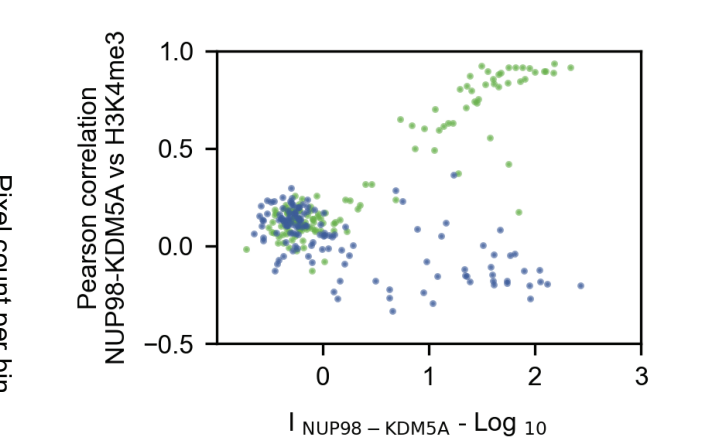
F NUP98-KDM5A-mEGFP; n = 134 NUP98-KDM5A-mut-mEGFP; n = 132
