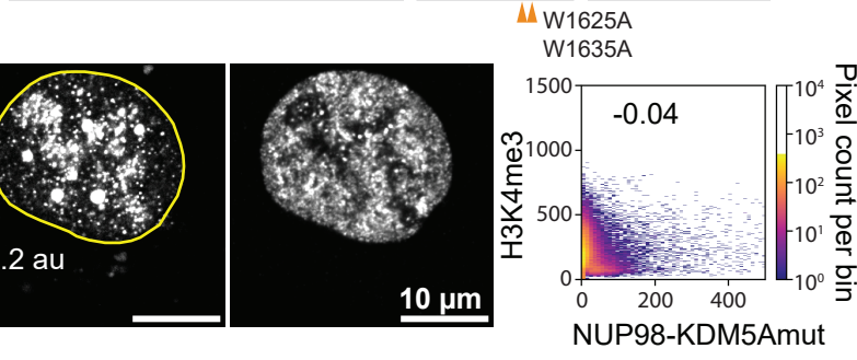
F NUP98-KDM5A-mEGFP; n = 134 NUP98-KDM5A-mut-mEGFP; n = 132
