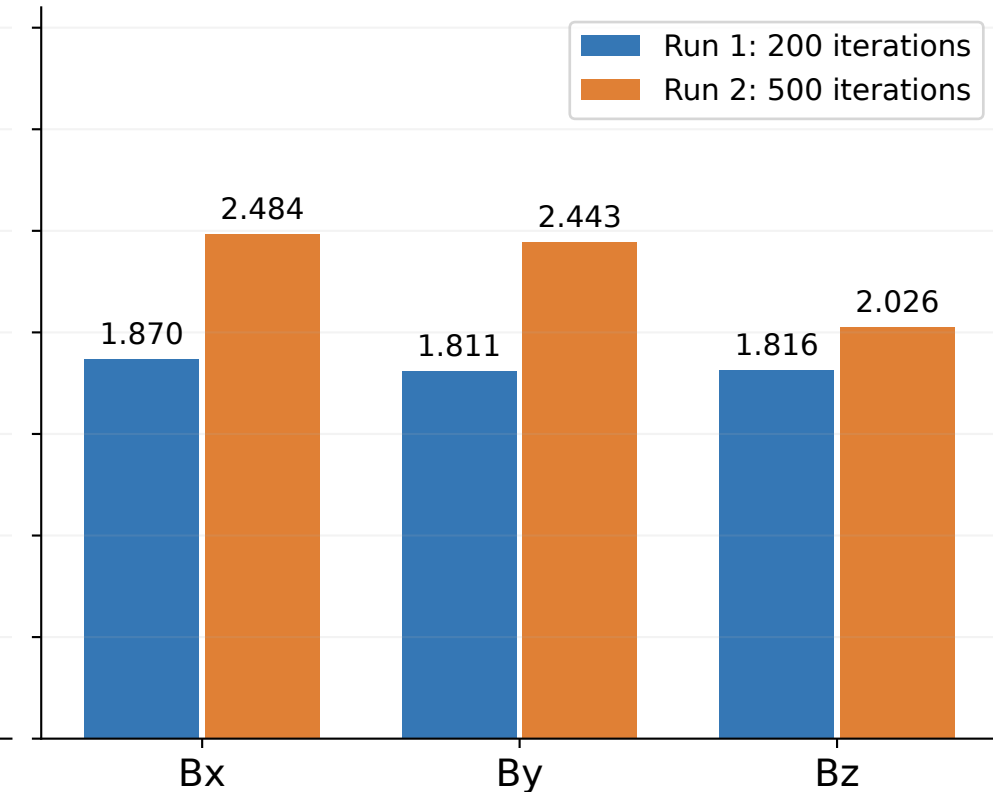
FISTA
