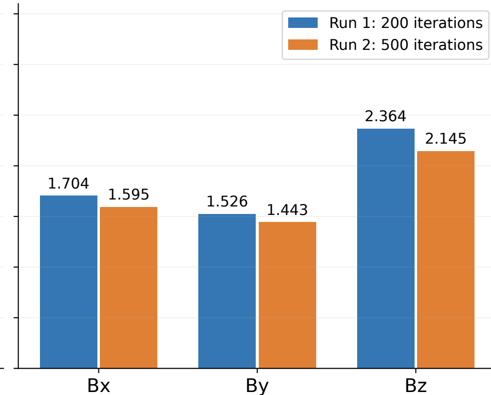
ISTA
