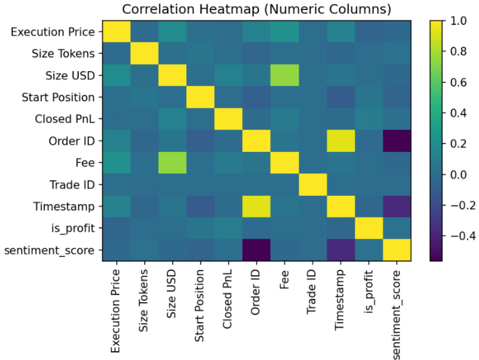
correlation_heatmap.png
