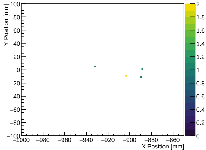
Deuterons: OMD Station 1 ( z \approx 25.6 m)
