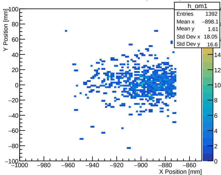
Off-Momentum Tracker Station 1 (Z ~ 25.6m)
