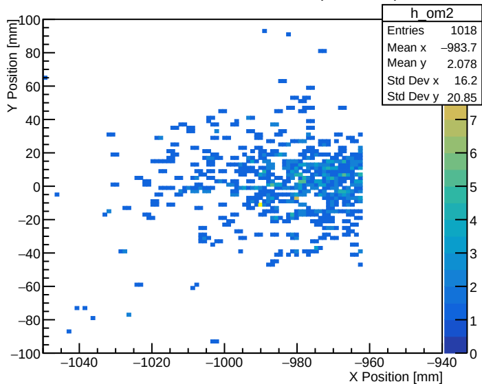
Off-Momentum Tracker Station 2 (Z ~ 26.9m)
