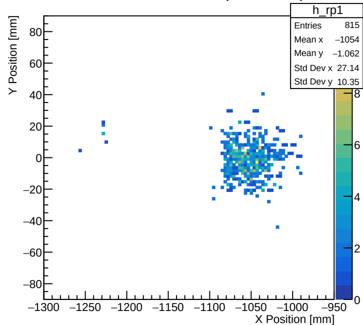
Roman Pot Station 1 (Z ~ 32.5m)
