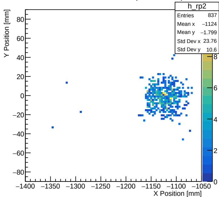
Roman Pot Station 2 (Z ~ 34.3m)
