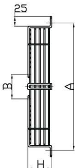
SIDE VIEW W/O FAN
