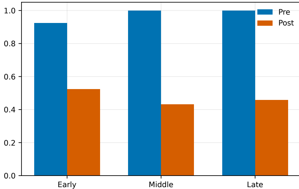
BFS
