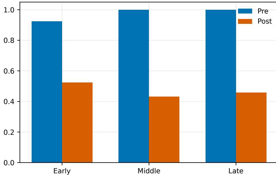
BFS
