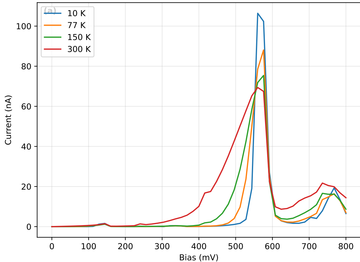
Mol A: I-V vs Temperature
