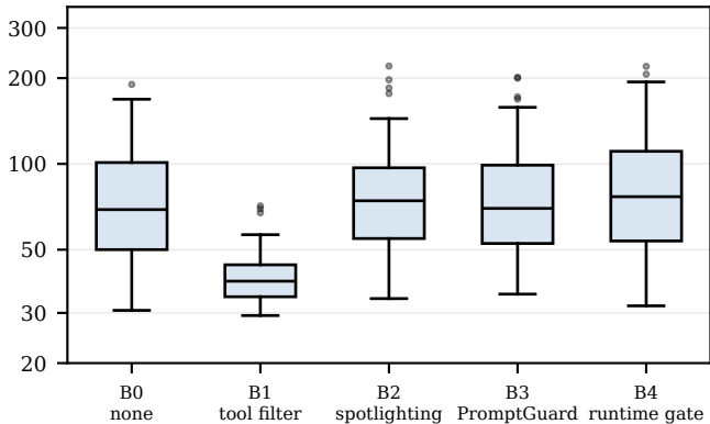
Qwen3-4B
