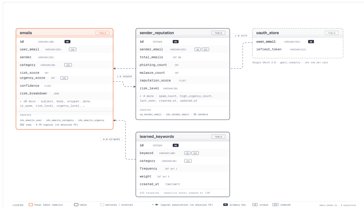
Figure 4.2: ER Diagram
