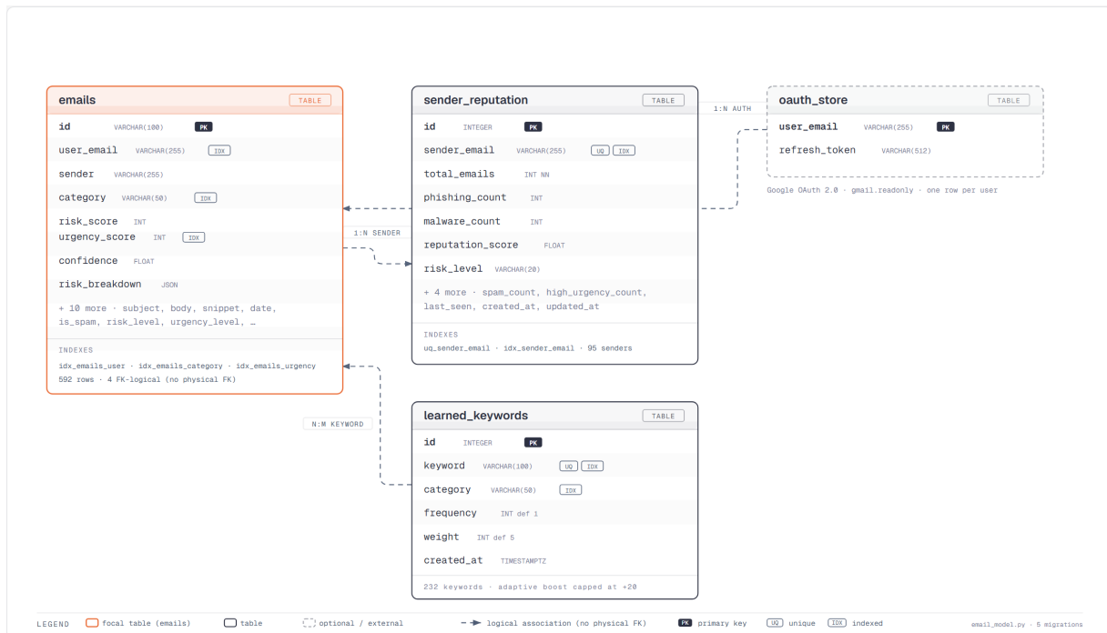
Figure 4.2: ER Diagram
