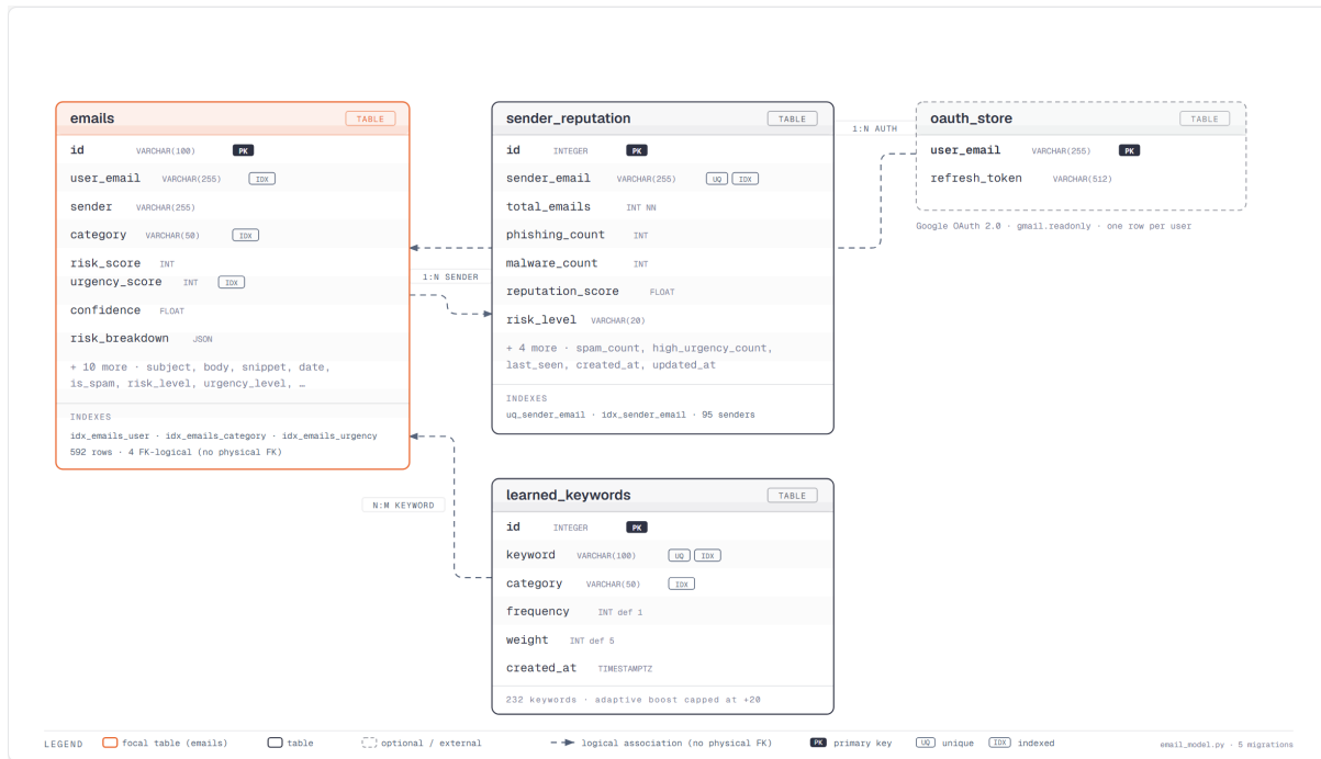
Figure 4.2: ER Diagram
