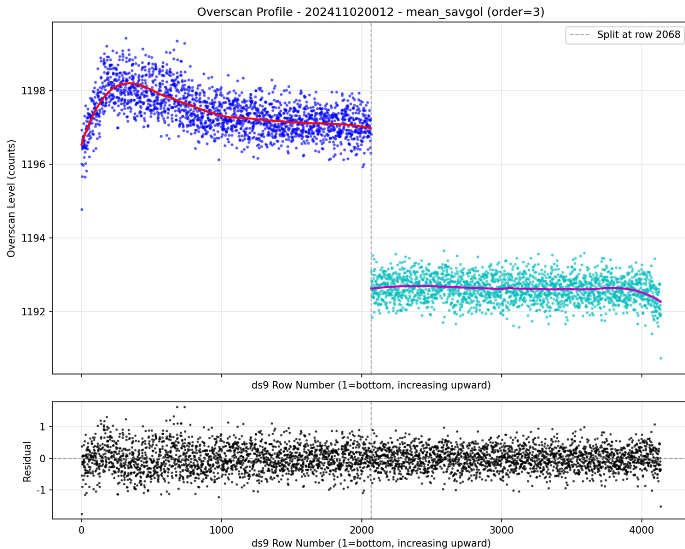
(图 2: 过扫区改正诊断图, 展示了单帧图像过扫区一维轮廓的拟合与扣除效果)
