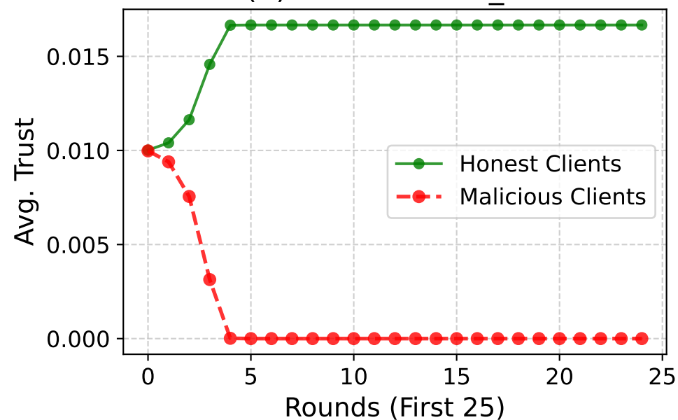
(b) MNIST - NON_IID
