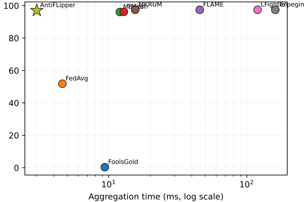
MNIST (IID)
