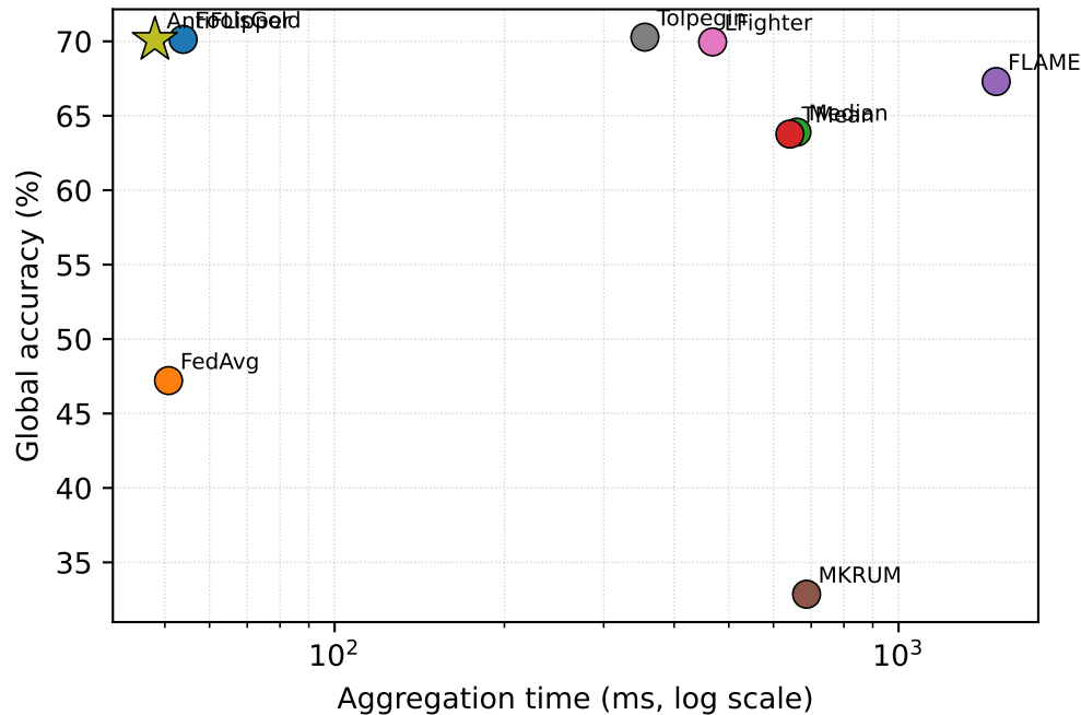
CIFAR-10 (IID)
