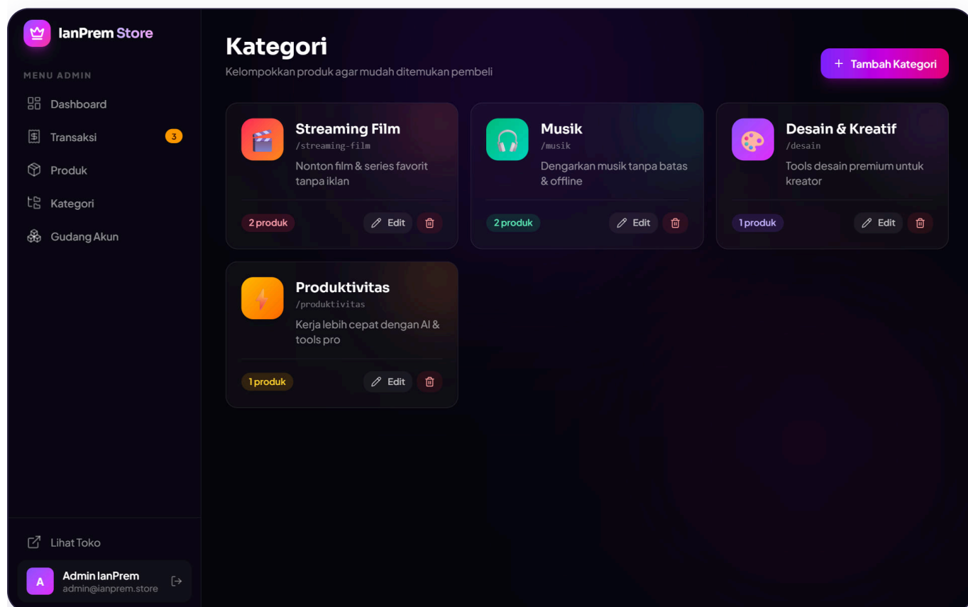
Gambar 6. Halaman Kategori
