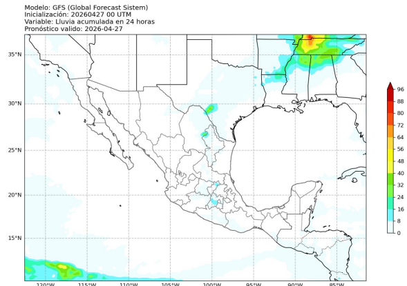
Figura 2: Pronóstico de lluvia acumulada (mm) a 24 horas (1 día). Válido hasta el 27 de abril de 2026 a las 06:00 p.m. Salida de modelo GFS.
