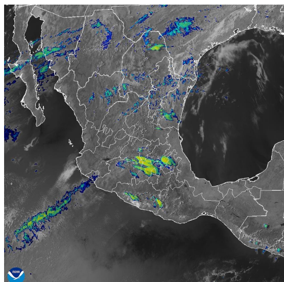
Figura 1. Imagen de satélite en canal infrarrojo obtenido del satélite GOES, 03:40 p.m. del Lunes 27 de abril de 2026.
