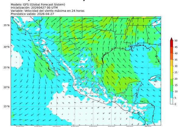
Figura 3: Pronóstico de comportamiento de viento a 10 metros a 24 horas (1 día). Válido hasta el 27 de abril de 2026 a las 06:00 p.m. Salida de modelo GFS.
