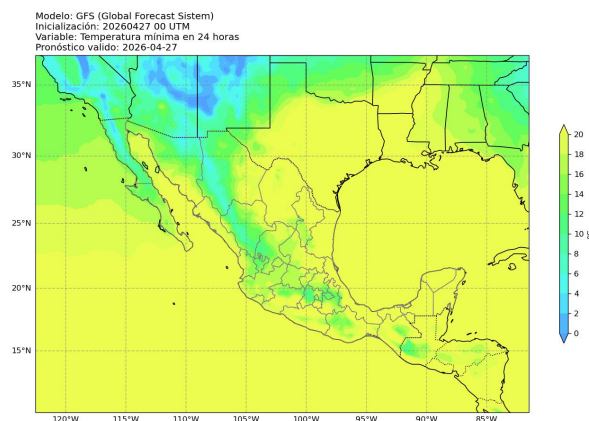
Figura 5: Pronóstico de temperatura mínima (°C) en 24 horas (1 día). Válido hasta el 27 de abril de 2026 a las 06:00 p.m. Salida de modelo GFS.
