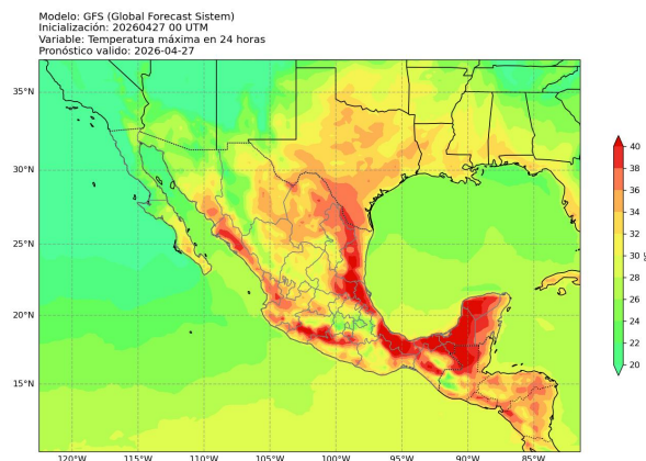
Figura 4: Pronóstico de temperatura máxima (°C) en 24 horas (1 día). Válido hasta el 27 de abril de 2026 a las 06:00 p.m. Salida de modelo GFS.
