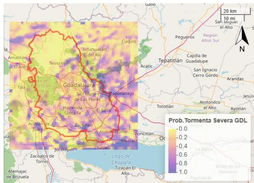
Figura 6: Pronóstico de desarrollo de tormentas para el 27 de abril de 2026 a las 06:00 p.m. Salida de modelo GFS.
