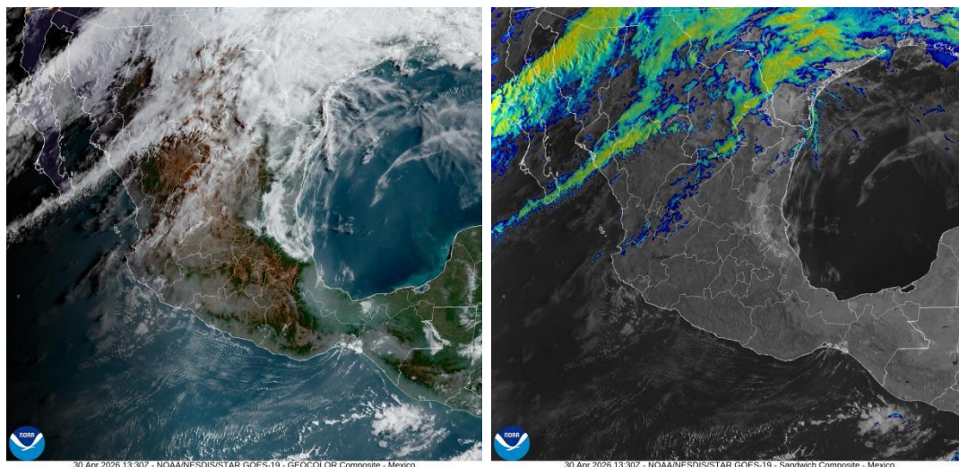
Figura 1. Imagen de satélite en canal luz visible (izquierda) e infrarrojo (derecha) obtenido del satélite GOES, 07:55 a.m. (hora local) del 30 de abril de 2026.
