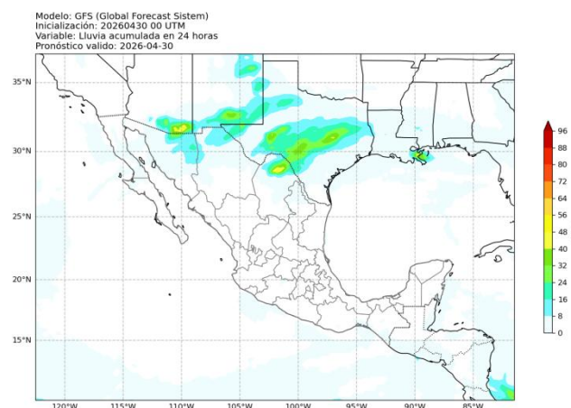
Figura 2: Pronóstico de lluvia acumulada (mm) a 24 horas. Válido hasta el 30 de abril de 2026 a las 08:00 a.m. (hora local). Salida de modelo GFS.
