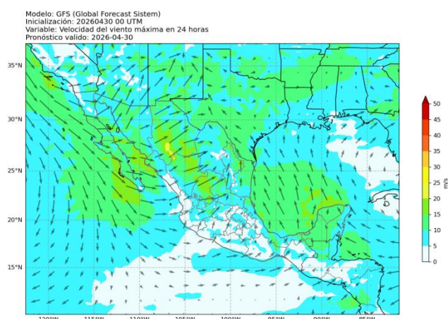
Figura 3: Pronóstico de viento a 10 metros a 24 horas. Válido hasta el 30 de abril de 2026 a las 08:00 a.m. (hora local). Salida de modelo GFS.
