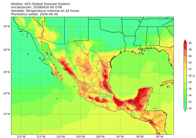
Figura 4: Pronóstico de temperatura máxima (°C) a 24 horas. Válido hasta el 30 de abril de 2026 a las 08:00 a.m. (hora local). Salida de modelo GFS.
