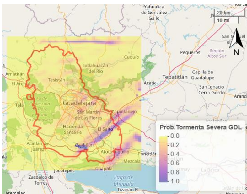
Figura 6: Pronóstico de desarrollo de tormentas para el 29 de abril de 2026. Consultado a las 08:00 am. del modelo GFS.
