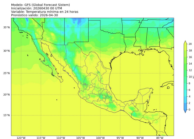
Figura 5: Pronóstico de temperatura mínima (°C) a 24 horas. Válido hasta el 30 de abril de 2026 a las 08:00 a.m. (hora local). Salida de modelo GFS.
