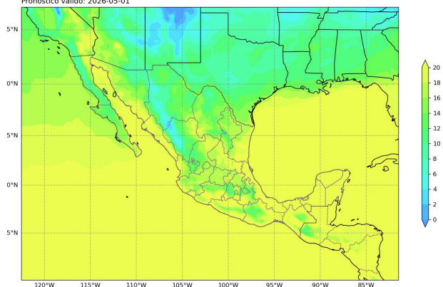
Figura 5: Pronóstico de temperatura mínima (°C) a 24 horas. Salida del modelo GFS para el 1 de mayo de 2026 a las 00 UTC. Consultado el 1 de mayo de 2026 a las 08:13 a.m.
