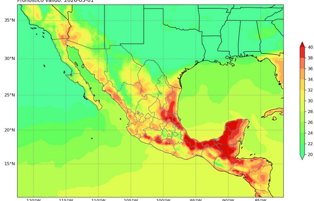
Figura 4: Pronóstico de temperatura máxima (°C) a 24 horas. Salida del modelo GFS para el 1 de mayo de 2026 a las 00 UTC. Consultado el 1 de mayo de 2026 a las 08:13 a.m.
