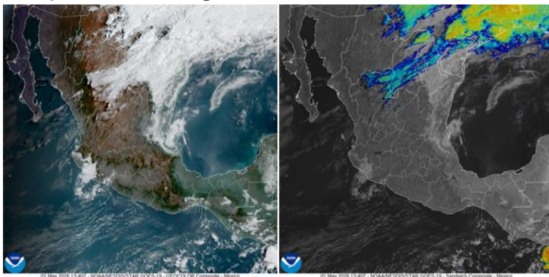
Figura 1. Imagen de satélite en canal luz visible (izquierda) e infrarrojo (derecha) obtenido del satélite GOES, 08:13 a.m. (hora local) del 01 de mayo de 2026.
