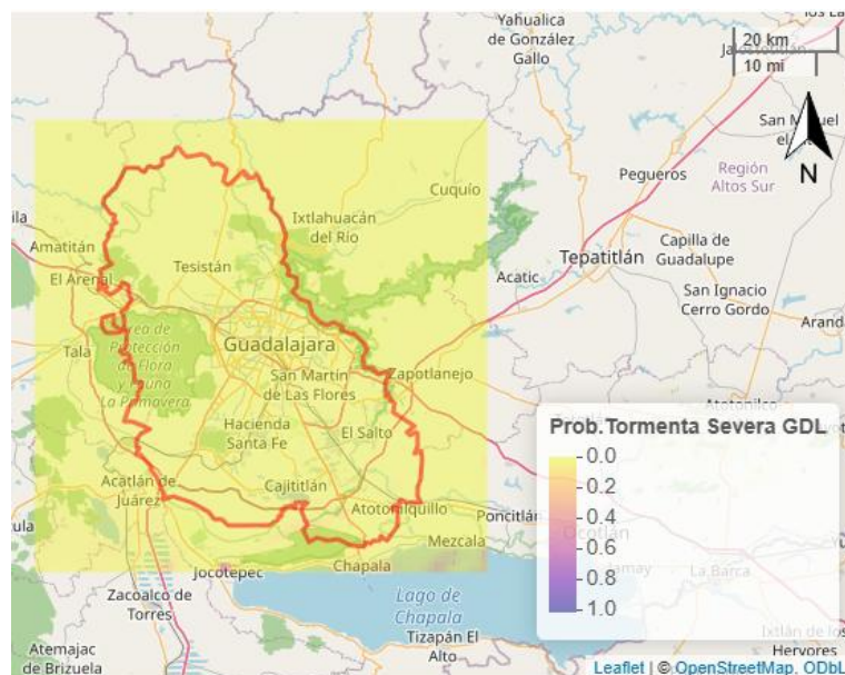
Figura 6: Pronóstico de desarrollo de tormentas para el 1 de mayo de 2026. Consultado a las 08:13 am. del modelo GFS.
