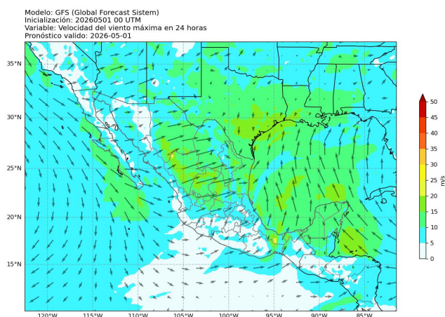
Figura 3: Pronóstico de viento a 10 metros a 24 horas. Salida del modelo GFS para el 1 de mayo de 2026 a las 00 UTC. Consultado el 1 de mayo de 2026 a las 08:13 a.m.
