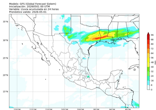
Figura 2: Pronóstico de lluvia acumulada (mm) a 24 horas. Salida del modelo GFS para el 1 de mayo de 2026 a las 00 UTC. Consultado el 1 de mayo de 2026 a las 08:13 a.m.
