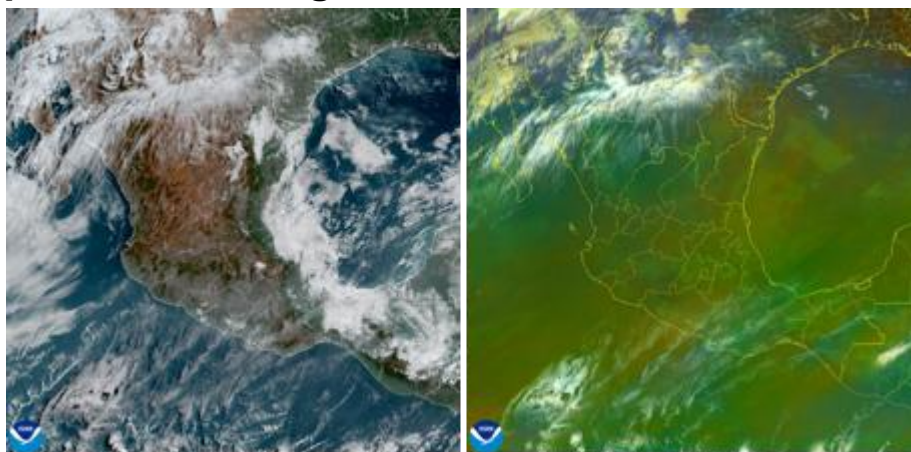
Figura 1. Imagen de satélite en canal luz visible (izquierda) e infrarrojo (derecha) obtenido del satélite GOES, 08:35 a.m. (hora local) del 04 de mayo de 2026.
