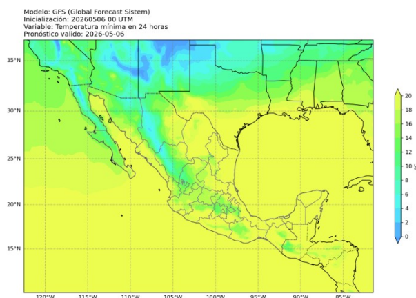
Figura 5: Pronóstico de temperatura mínima (°C) a 24 horas. Salida del modelo GFS para el 6 de mayo de 2026 a las 00 UTC. Consultado el 6 de mayo de 2026 a las 08:32 hrs.
