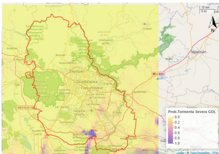
Figura 6: Pronóstico de desarrollo de tormentas para el 6 de mayo de 2026. Consultado a las 08:32 a.m. [hora local] del modelo GFS.
