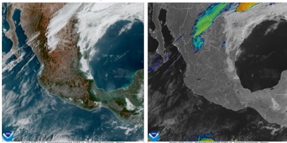
Figura 1. Imagen de satélite en canal luz visible (izquierda) e infrarrojo (derecha) obtenido del satélite GOES, 08:35 a.m. (hora local) del 05 de mayo de 2026.
