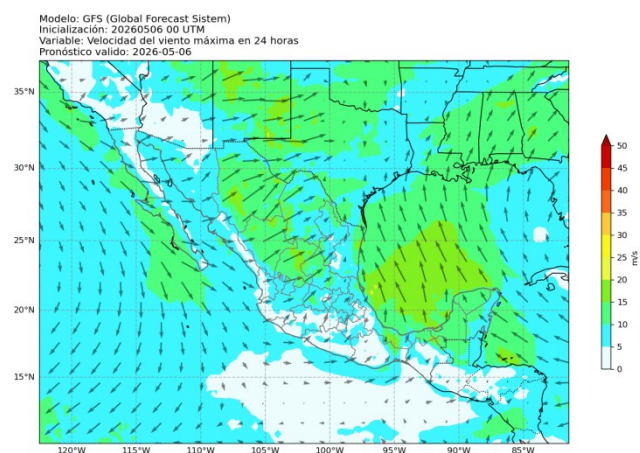
Figura 3: Pronóstico de viento a 10 metros a 24 horas. Salida del modelo GFS para el 6 de mayo de 2026 a las 00 UTC. Consultado el 6 de mayo de 2026 a las 08:32 hrs.
