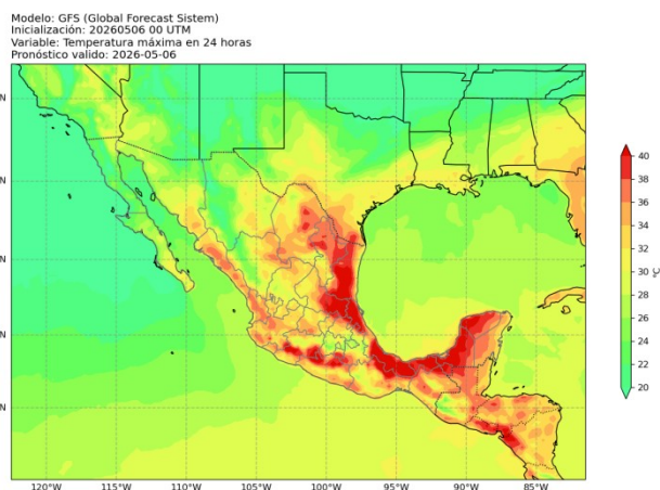
Figura 4: Pronóstico de temperatura máxima (°C) a 24 horas. Salida del modelo GFS para el 6 de mayo de 2026 a las 00 UTC. Consultado el 6 de mayo de 2026 a las 08:32 hrs.
