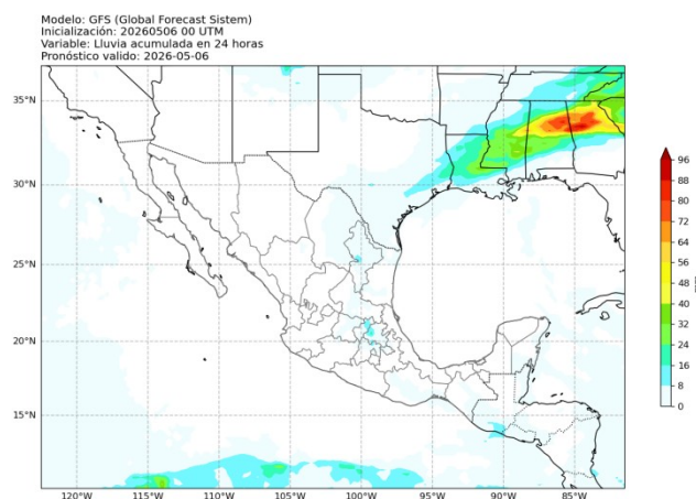
Figura 2: Pronóstico de lluvia acumulada (mm) a 24 horas. Salida del modelo GFS para el 6 de mayo de 2026 a las 00 UTC. Consultado el 6 de mayo de 2026 a las 08:32 hrs.
