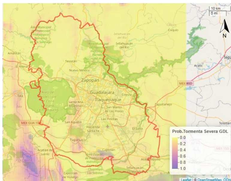
Figura 6: Pronóstico de desarrollo de tormentas para el 07 de mayo de 2026. Consultado a las 08:19 a.m. (hora local) desde el modelo GFS.
