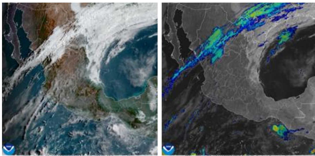
Figura 1. Imagen de satélite en canal luz visible (izquierda) e infrarrojo (derecha) obtenido del satélite GOES, 08:13 a.m. (hora local) del 07 de mayo de 2026.
