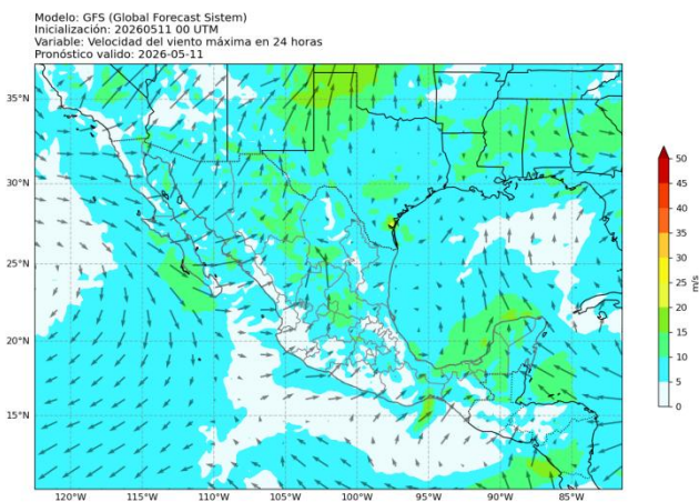
Figura 3: Pronóstico de viento a 10 metros a 24 horas. Salida del modelo GFS para el 11 de mayo de 2026 a las 00 UTC. Consultado el 11 de mayo de 2026 a las 08:37 hrs.
