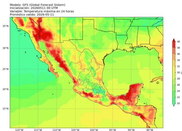
Figura 4: Pronóstico de temperatura máxima (°C) a 24 horas. Salida del modelo GFS para el 11 de mayo de 2026 a las 00 UTC. Consultado el 11 de mayo de 2026 a las 08:37 hrs.
