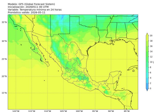
Figura 5: Pronóstico de temperatura mínima (°C) a 24 horas. Salida del modelo GFS para el 11 de mayo de 2026 a las 00 UTC. Consultado el 11 de mayo de 2026 a las 08:37 hrs.
