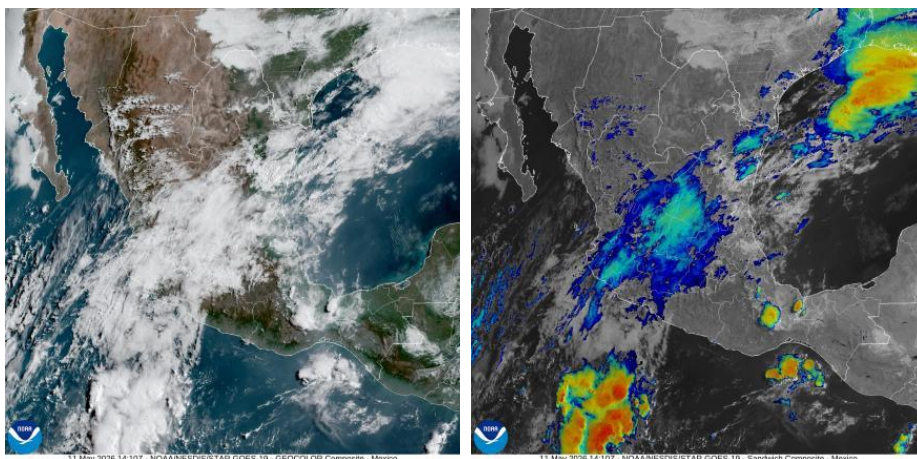
Figura 1. Imagen de satélite en canal luz visible (izquierda) e infrarrojo (derecha) obtenido del satélite GOES, 08:37 a.m. (hora local) del 11 de mayo de 2026.
