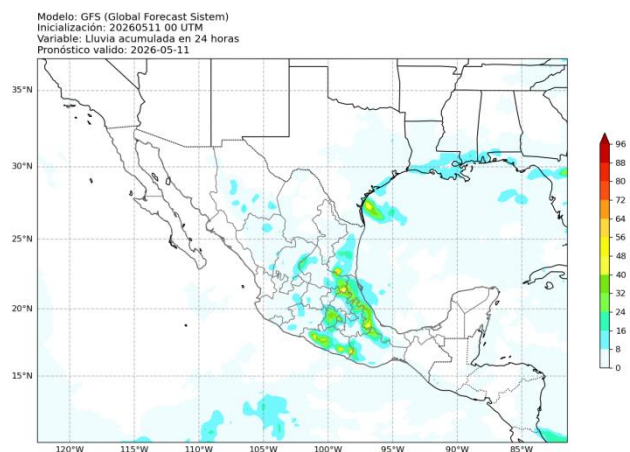
Figura 2: Pronóstico de lluvia acumulada (mm) a 24 horas. Salida del modelo GFS para el 11 de mayo de 2026 a las 00 UTC. Consultado el 11 de mayo de 2026 a las 08:37 hrs.
