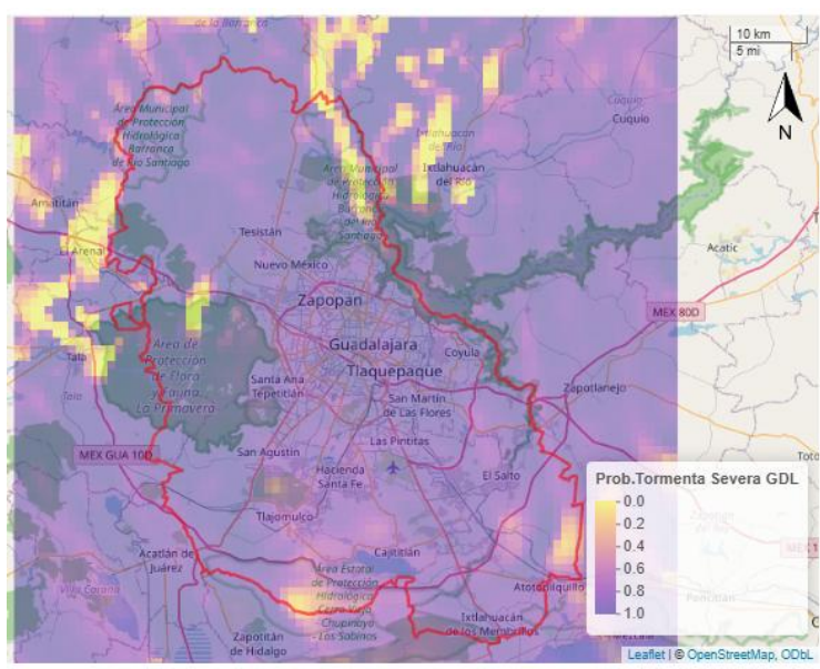
Figura 6: Pronóstico de desarrollo de tormentas para el 11 de mayo de 2026. Consultado a las 08:17 a.m. (hora local) desde el modelo GFS.
