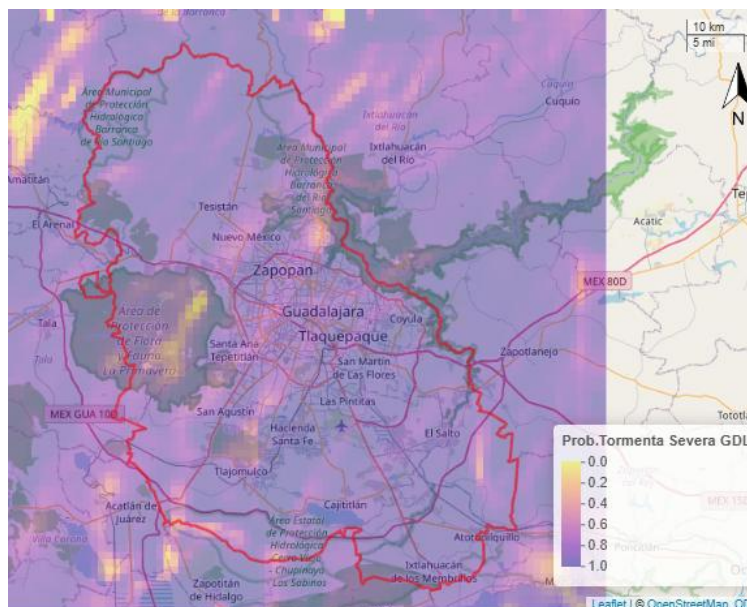
Figura 6: Pronóstico de desarrollo de tormentas para el 12 de mayo de 2026. Consultado a las 08:47 a.m. (hora local) desde el modelo GFS.
