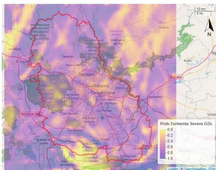
Figura 6: Pronóstico de desarrollo de tormentas para el 14 de mayo de 2026. Consultado a las 08:35 a.m. (hora local) desde el modelo GFS.
