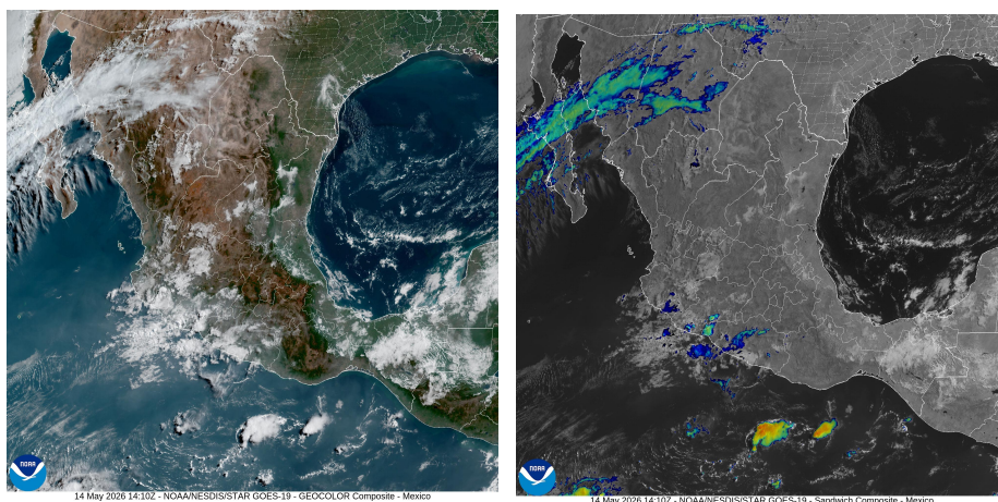
Figura 1. Imagen de satélite en canal luz visible (izquierda) e infrarrojo (derecha) obtenido del satélite GOES, 08:00 a.m. (hora local) del 14 de mayo de 2026.
