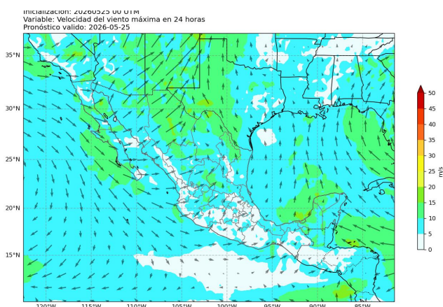
Figura 3: Velocidad del viento (m/s) pronosticada a 24 horas. Modelo WRF (inicializado con GFS). Válido para el 25 de mayo de 2026, 00 UTC.
