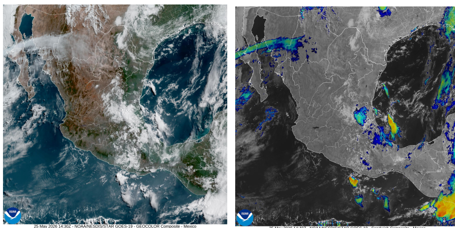
Figura 1. Imagen de satélite en canal luz visible (izquierda) e infrarrojo (derecha) obtenido del satélite GOES, 08:00 a.m. (hora local) del 25 de mayo de 2026.
