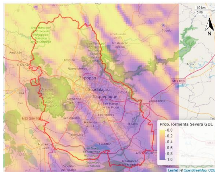
Figura 6: Pronóstico de desarrollo de tormentas para el 25 de mayo de 2026. Consultado a las 09:00 a.m. (hora local) desde el modelo GFS.
