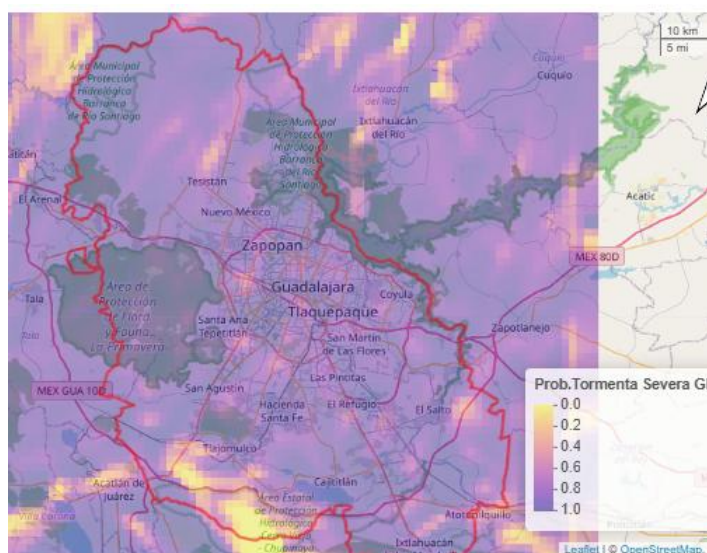
Figura 6: Pronóstico de desarrollo de tormentas para el 03 de junio de 2026. Consultado a las 09:00 a.m. (hora local) desde el modelo GFS.
