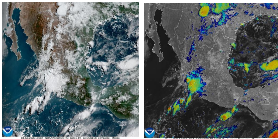
Figura 1. Imagen de satélite en canal luz visible (izquierda) e infrarrojo (derecha) obtenido del satélite GOES, 08:00 a.m. (hora local) del 03 de junio de 2026.
