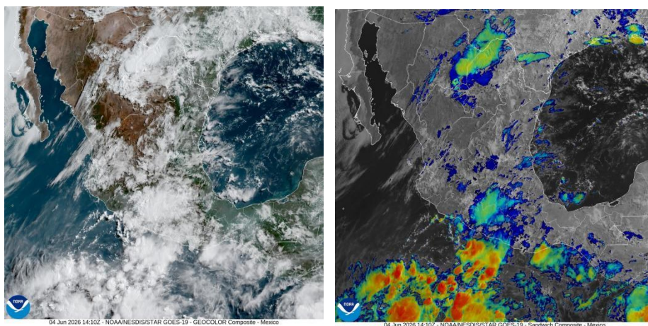
Figura 1. Imagen de satélite en canal luz visible (izquierda) e infrarrojo (derecha) obtenido del satélite GOES, 08:00 a.m. (hora local) del 04 de junio de 2026.
