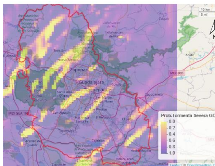
Figura 6: Pronóstico de desarrollo de tormentas para el 04 de junio de 2026. Consultado a las 09:00 a.m. (hora local) desde el modelo
