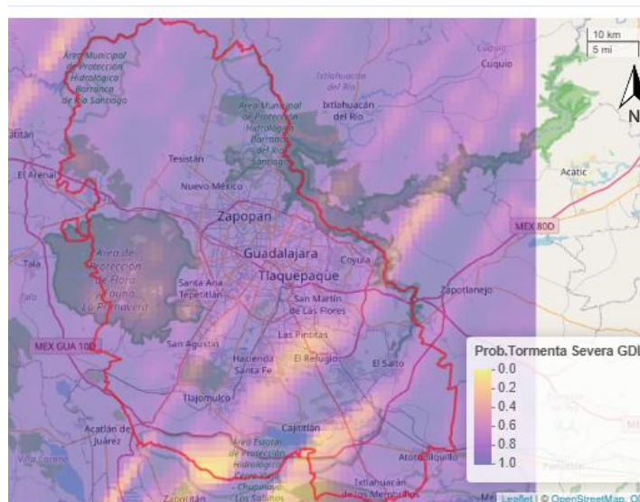
Figura 6: Pronóstico de desarrollo de tormentas para el 05 de junio de 2026. Consultado a las 09:00 a.m. (hora local) desde el modelo
