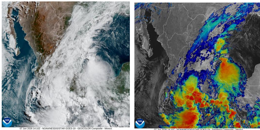
Figura 1. Imagen de satélite en canal luz visible (izquierda) e infrarrojo (derecha) obtenido del satélite GOES, 08:00 a.m. (hora local) del 07 de junio de 2026.
