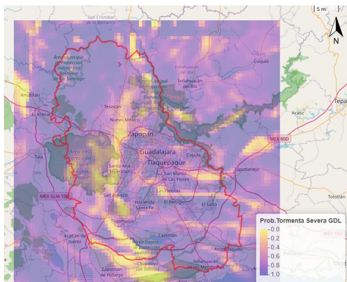
Figura 6: Pronóstico de desarrollo de tormentas para el 07 de junio de 2026. Consultado a las 09:00 a.m. (hora local) desde el modelo GFS.
