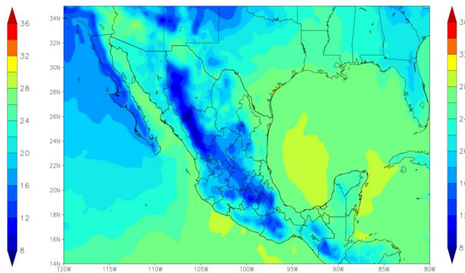
Figura 5: Temperatura mínima (°C) pronosticada a 24 horas. Modelo WRF (inicializado con GFS). Válido para el 08 de junio de 2026, 00 UTC.
