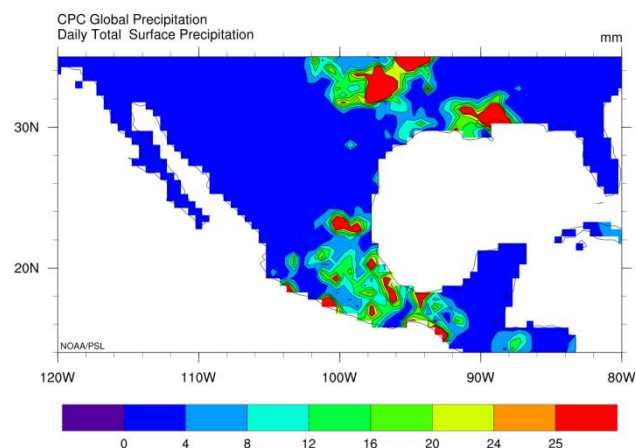
Figura 2: Lluvia acumulada (mm) a 24 horas. Fuente: NOAA Climate Prediction Center (CPC) / [07/jun/2026]. Válido para el 08 de junio de 2026, 00 UTC.
