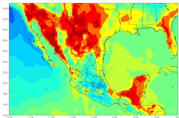
Figura 4: Temperatura máxima (°C) pronosticada a 24 horas. Modelo WRF (inicializado con GFS). Válido para el 08 de junio de 2026, 00 UTC.
