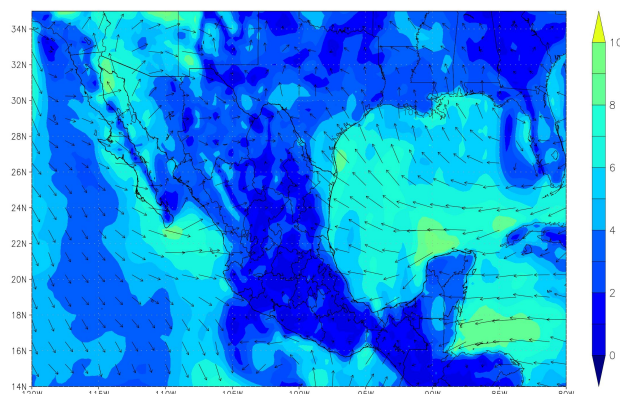
Figura 3: Velocidad del viento (m/s) en 24 horas. Elaboración propia con datos de ERA5 (Copernicus) y software GrADS. Válido para el 08 de junio de 2026, 00 UTC.
