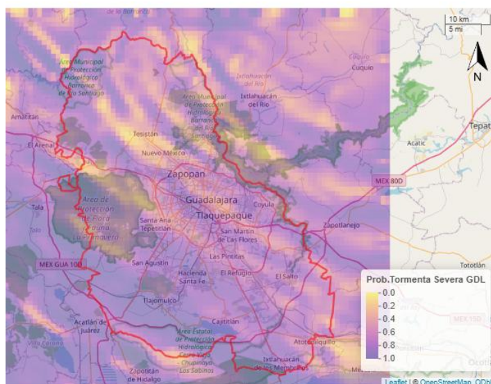
Figura 6: Pronóstico de desarrollo de tormentas para el 08 de junio de 2026. Consultado a las 09:00 a.m. (hora local) desde el modelo
