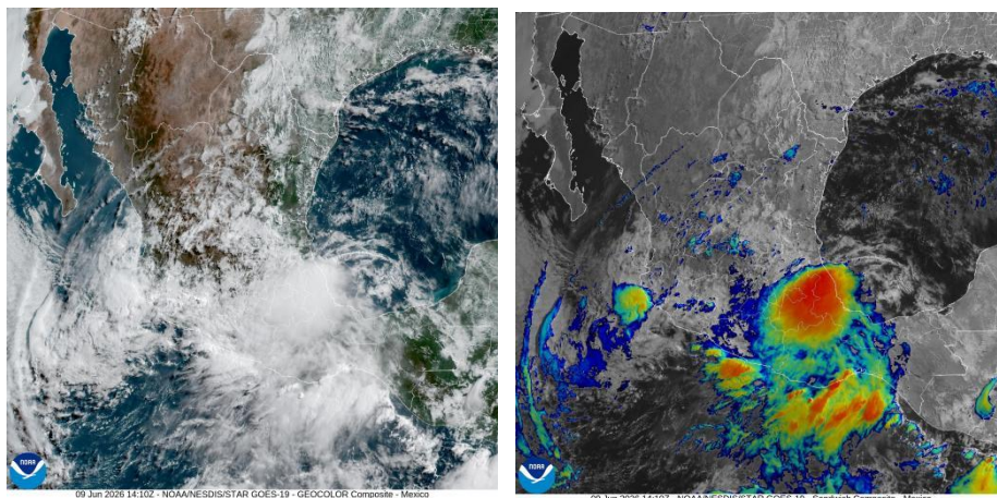
Figura 1. Imagen de satélite en canal luz visible (izquierda) e infrarrojo (derecha) obtenido del satélite GOES, 08:00 a.m. (hora local) del 09 de junio de 2026.
